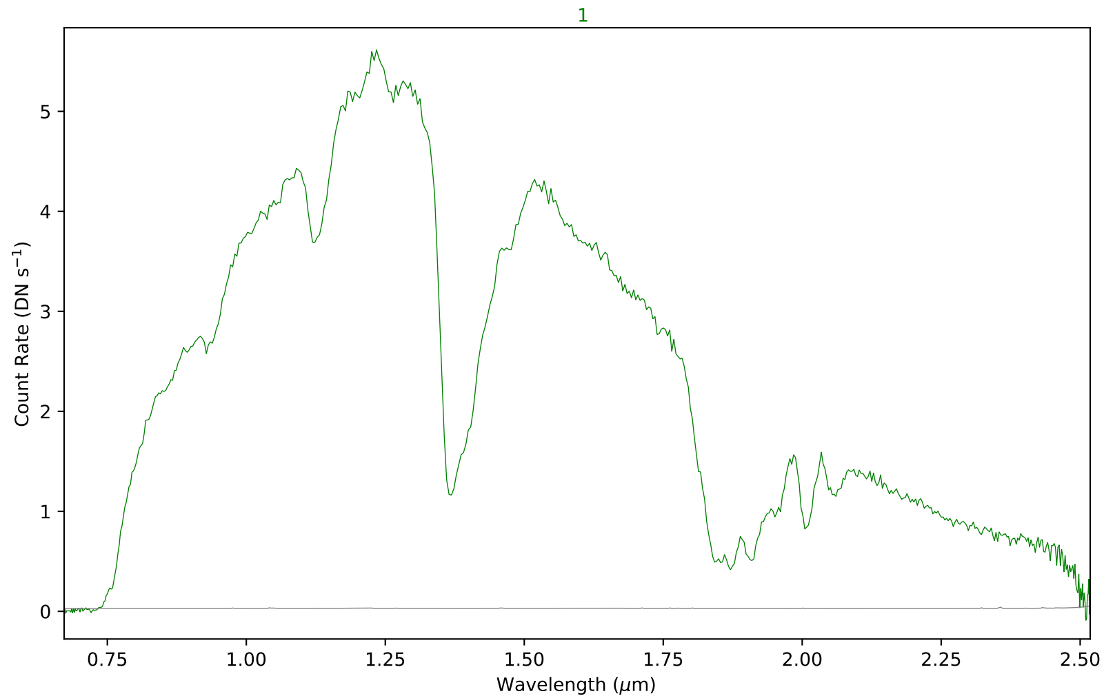
combspec2185-2200.fits - Aperture 1
