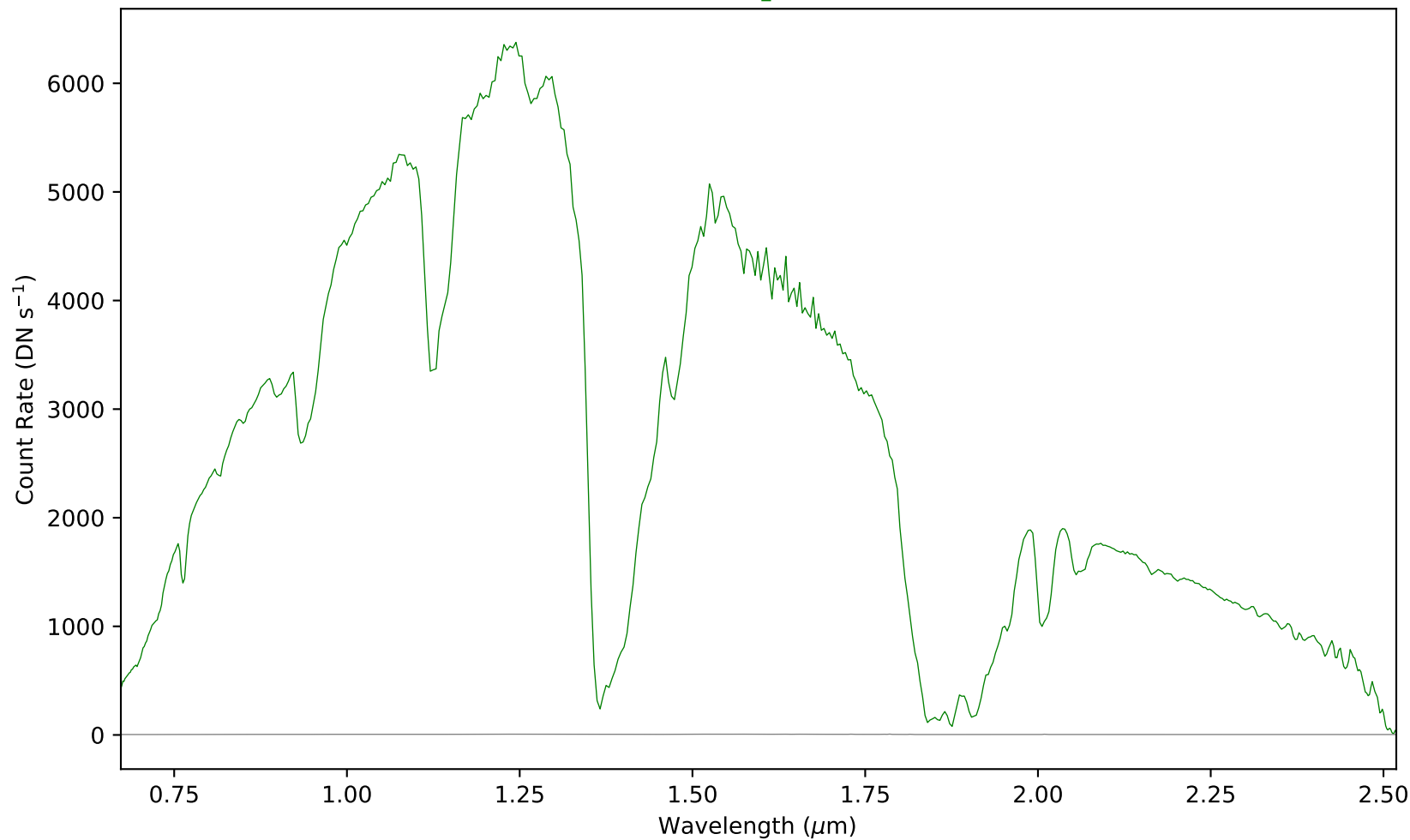
combspec185-190.fits - Aperture 1
