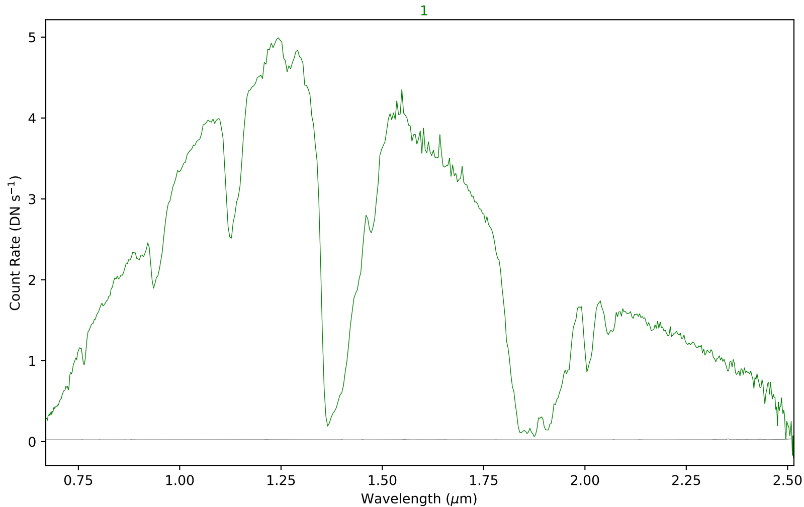
combspec339-358.fits - Aperture 1
