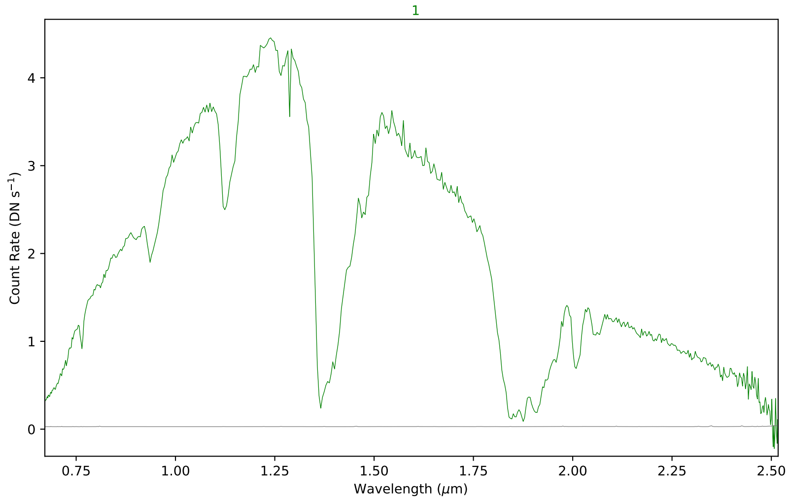
combspec801-830.fits - Aperture 1
