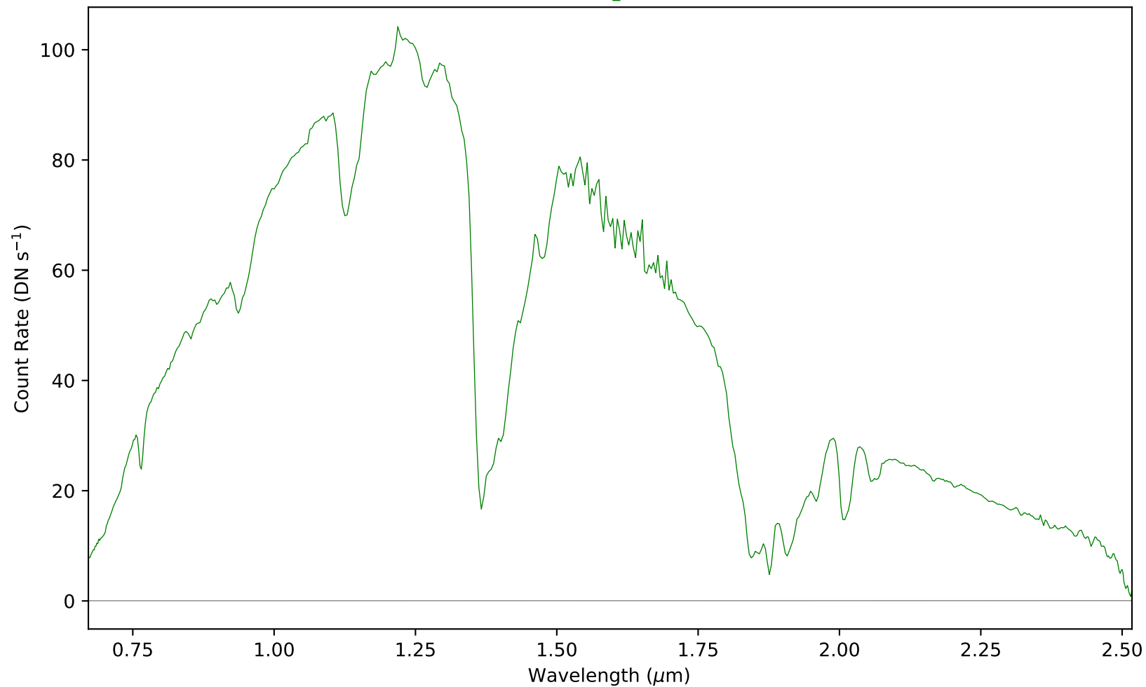
combspec234-247.fits - Aperture 1
