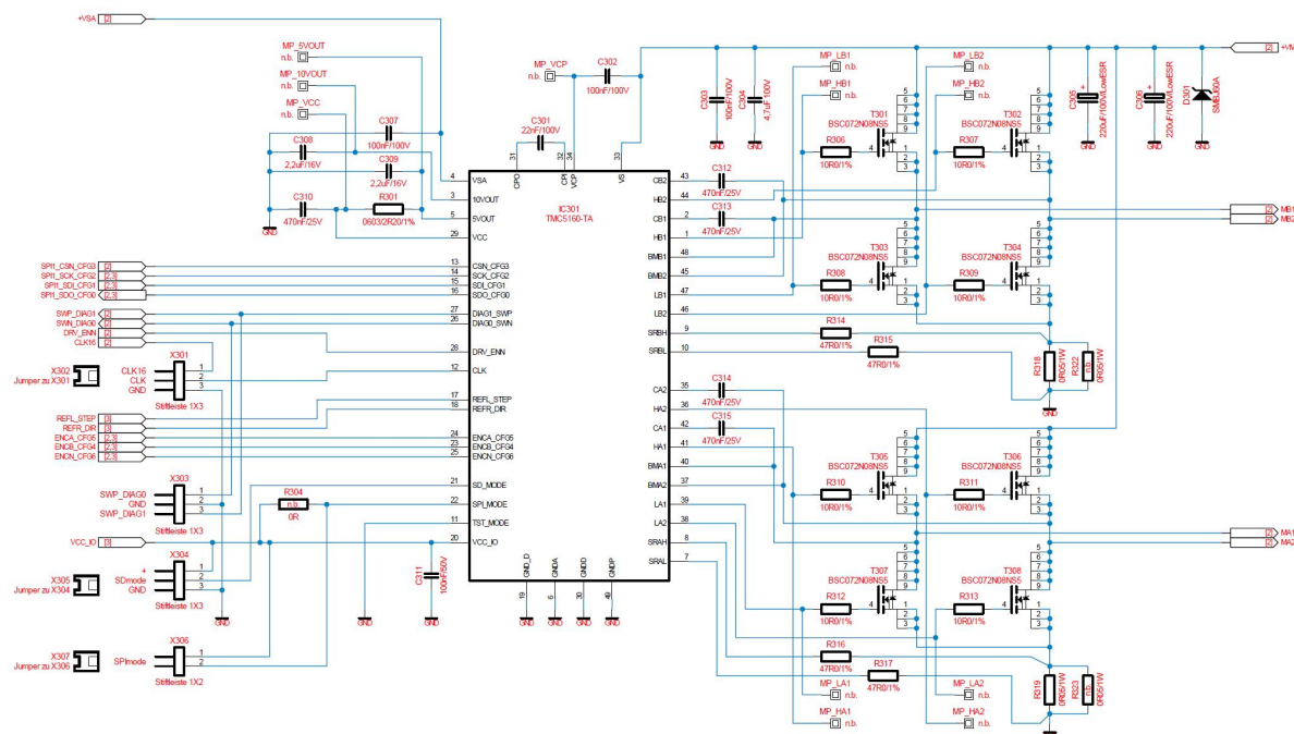
原理图(TMC5160+MOSFETs)
