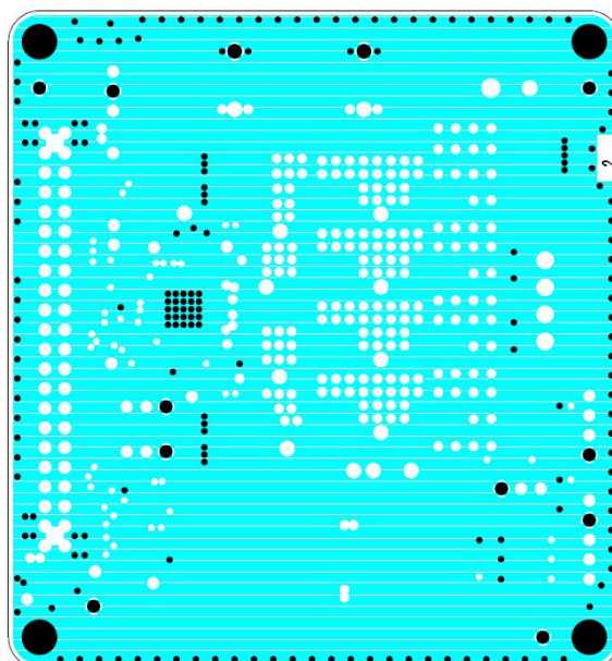
2- 内层(地)
