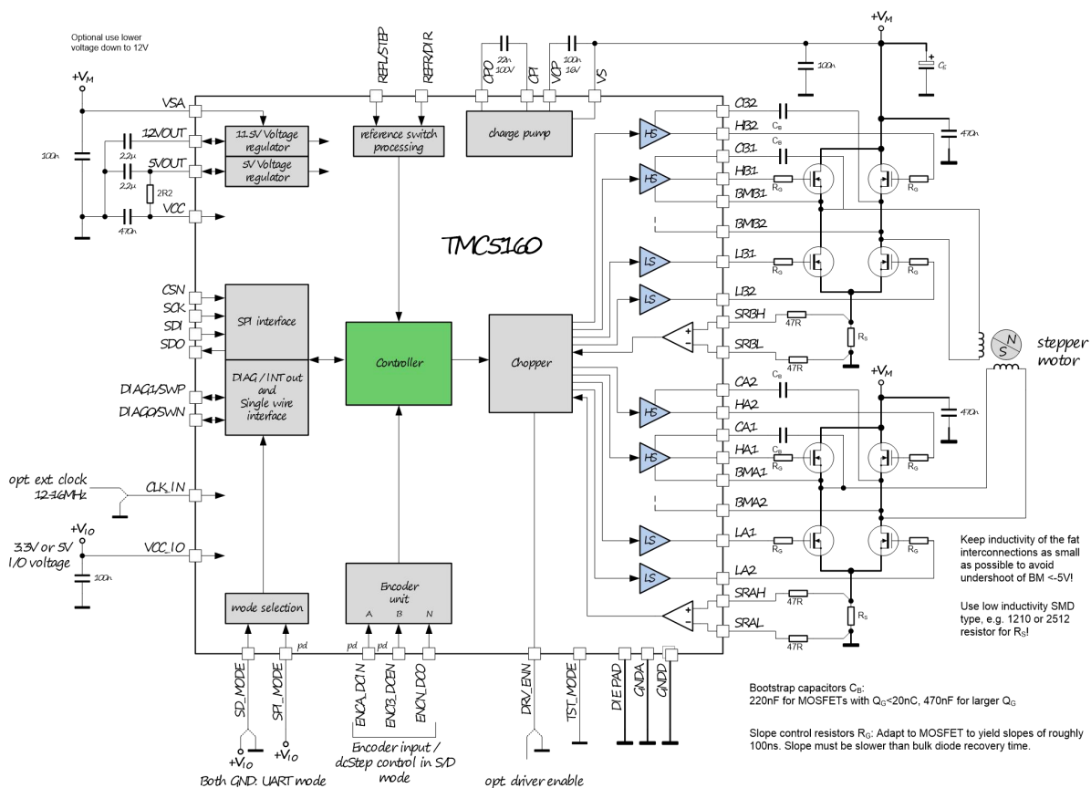
图 3.1 标准电路
