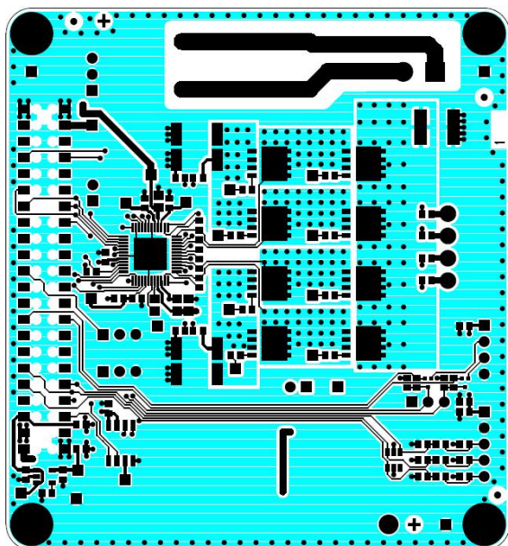
1- 顶层 (焊接側)
