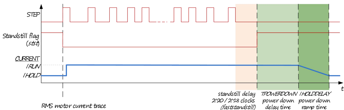
图 1.4 电机自动降电流
