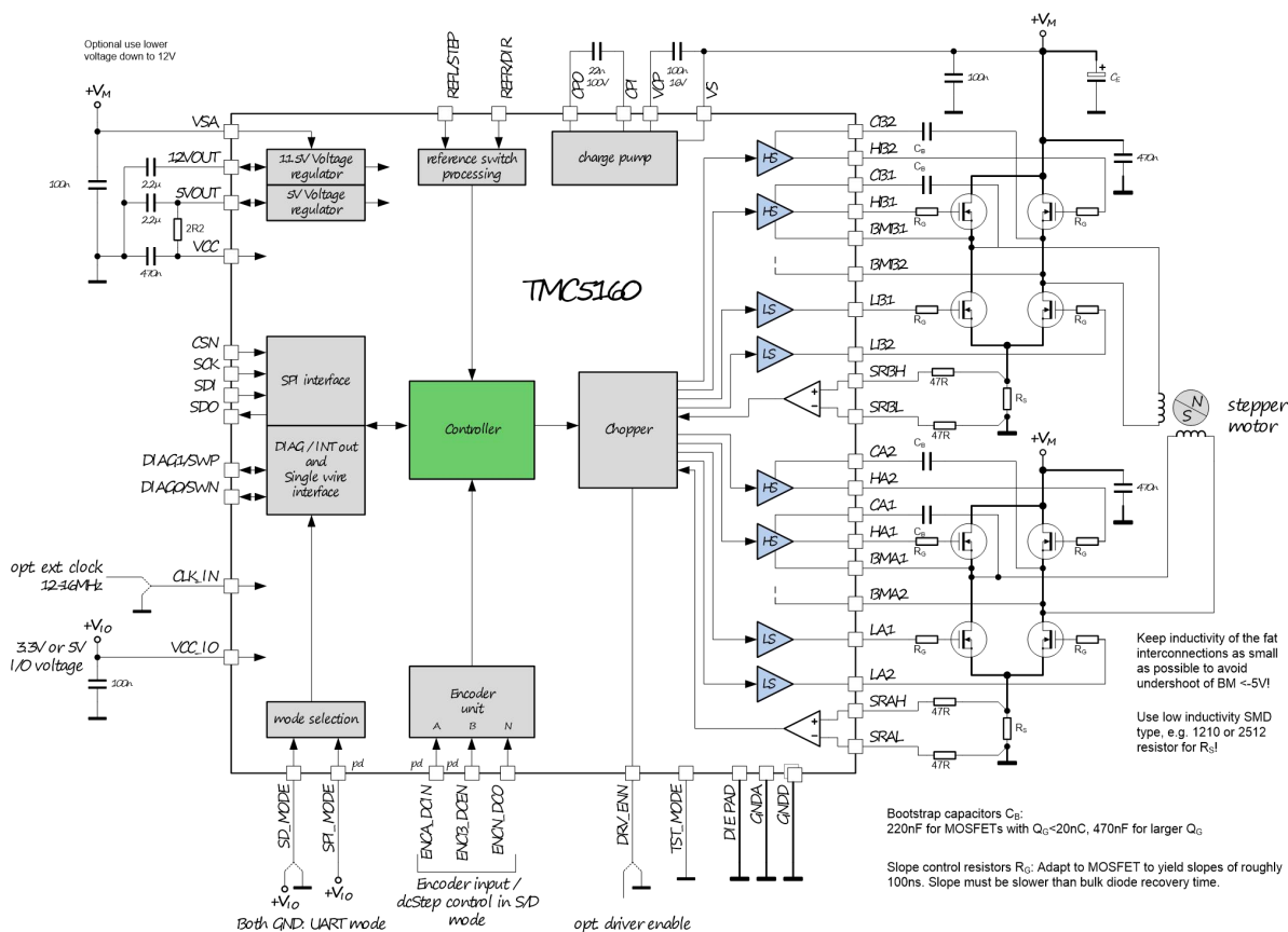
图 3.1 标准电路
