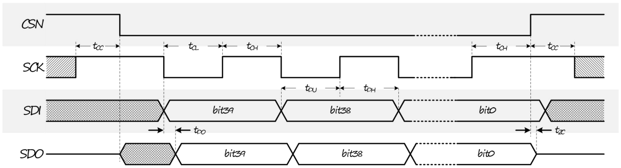
图 4.1 SPI 时序
