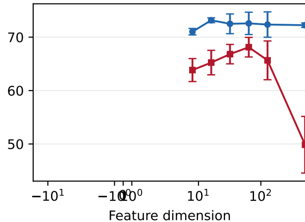
KMNIST
