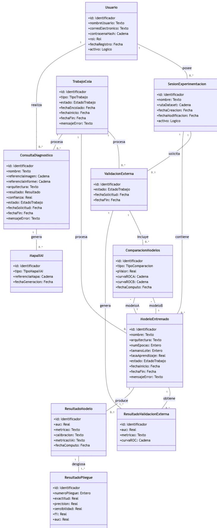
Ilustración 21 - Diagrama de clases del sistema
