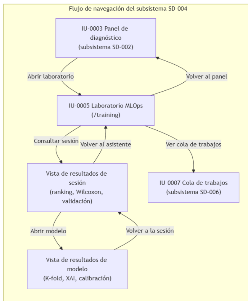
Ilustración 80 - Flujo de navegación del subsistema SD-004
