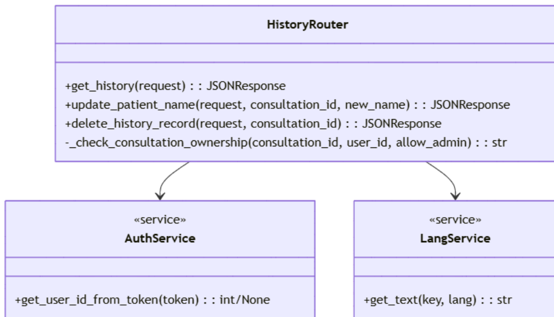
Ilustración 72 - Diagrama de clases del subsistema SD-003
