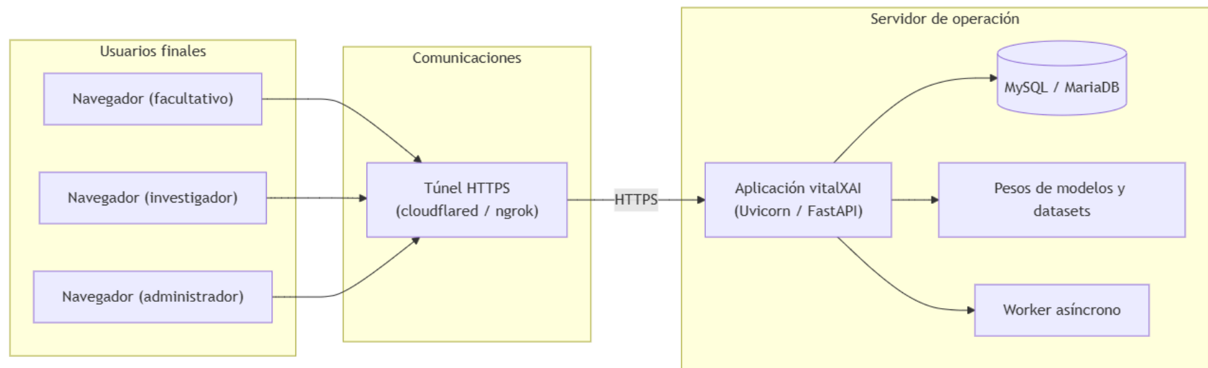
Ilustración 89 - Diagrama de implantación del sistema en el entorno de operación
