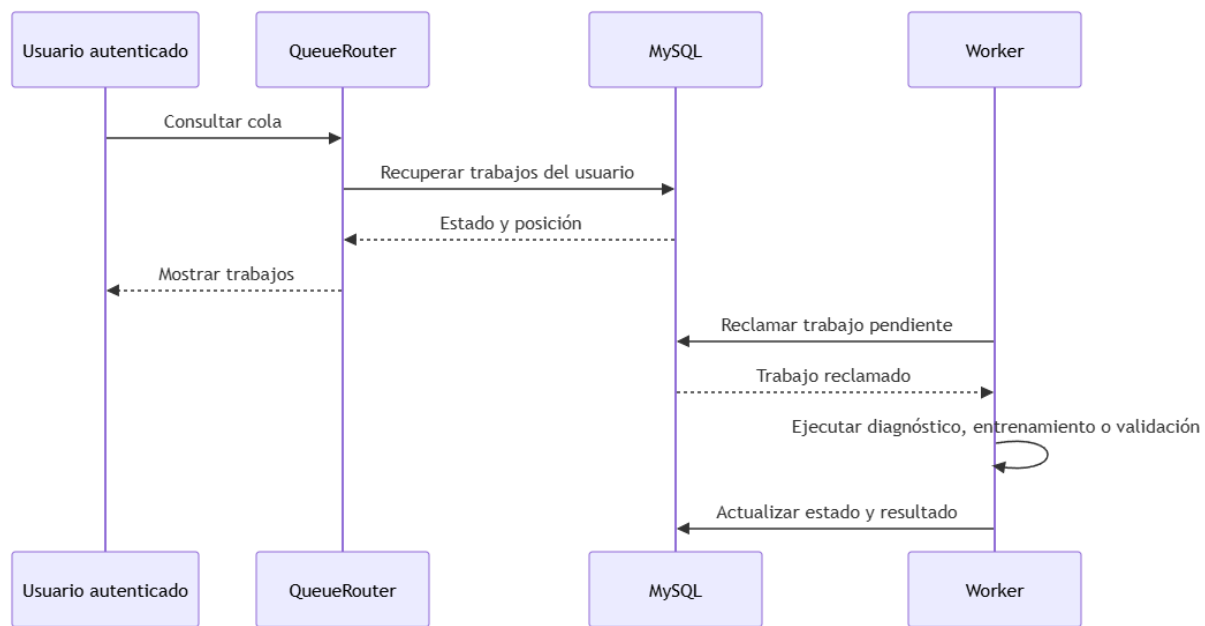
Ilustración 69 - SD-006: Cola de trabajos y capacidades transversales
