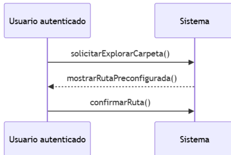
Ilustración 39 - Secuencia de interacción de la selección de la carpeta del dataset (CU-017)
