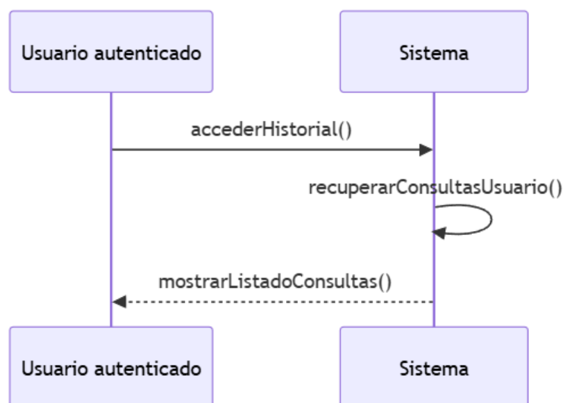
Ilustración 33 - Secuencia de interacción de la consulta del historial (CU-011)
