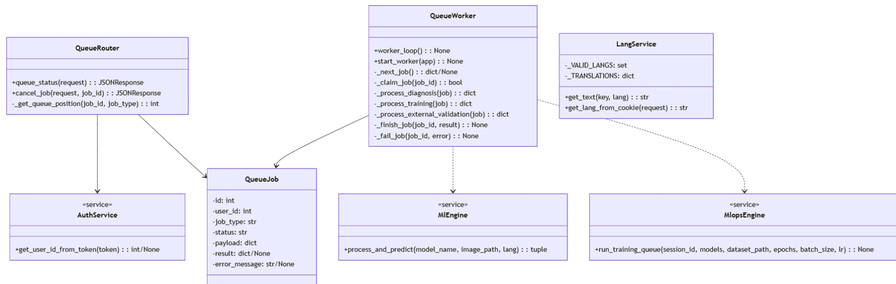
Ilustración 75 - Diagrama de clases del subsistema SD-006
