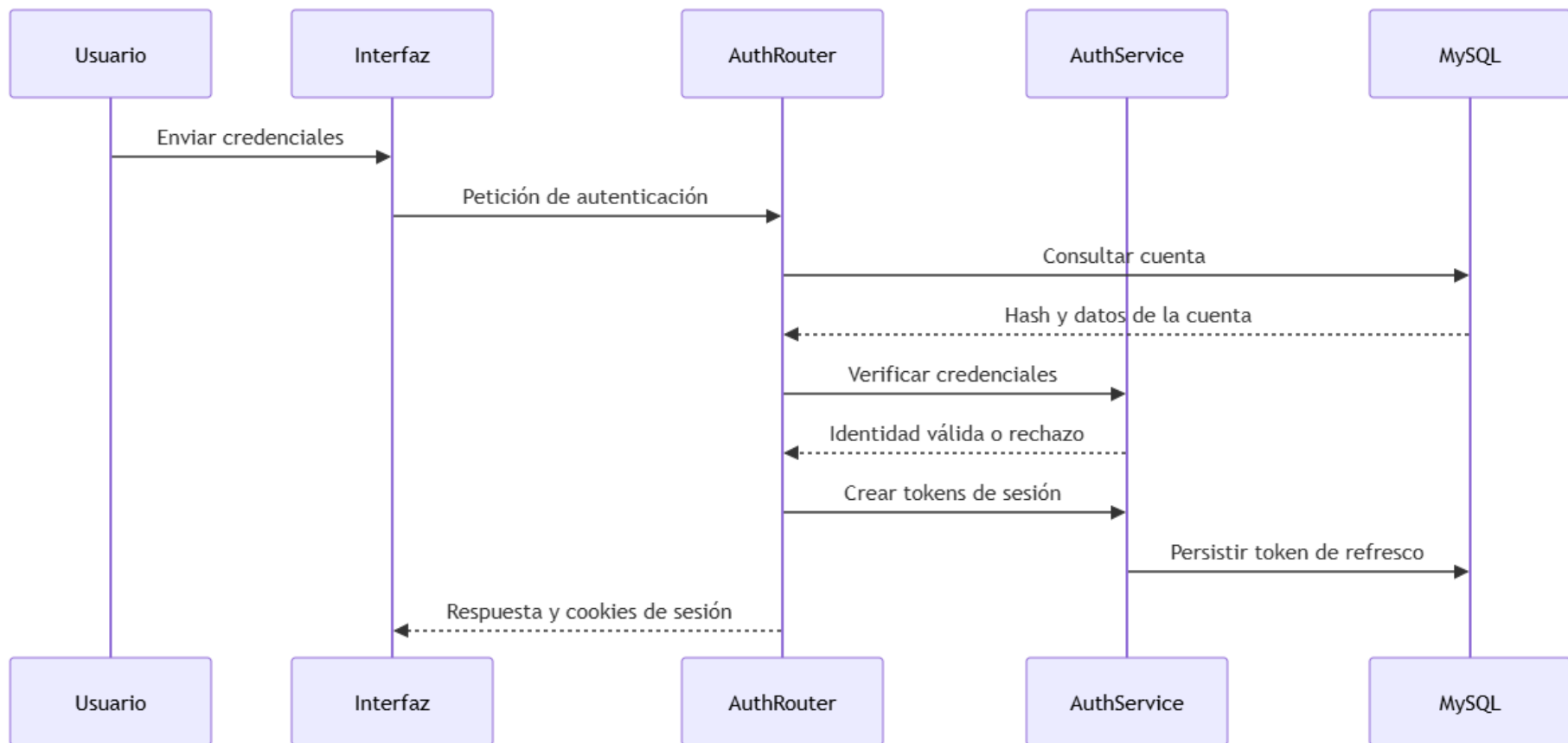
Ilustración 64 - SD-001: Acceso, identidad y gestión de sesiones
