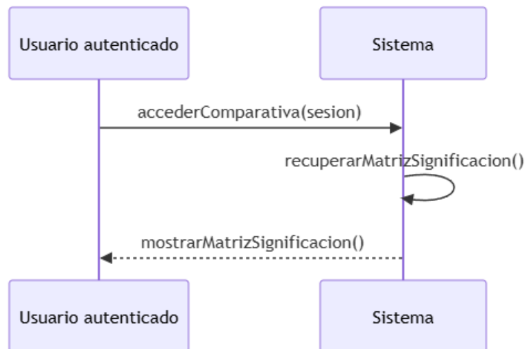
Ilustración 45 - Secuencia de interacción de la consulta de la comparativa estadística (CU-023)
