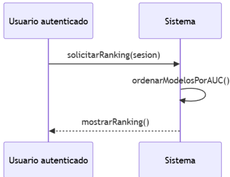
Ilustración 44 - Secuencia de interacción de la consulta del ranking (CU-022)
