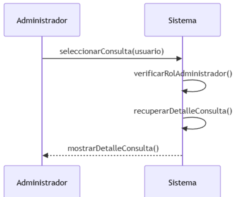
Ilustración 56 - Secuencia de interacción de la visualización del detalle de una consulta (CU-033)
