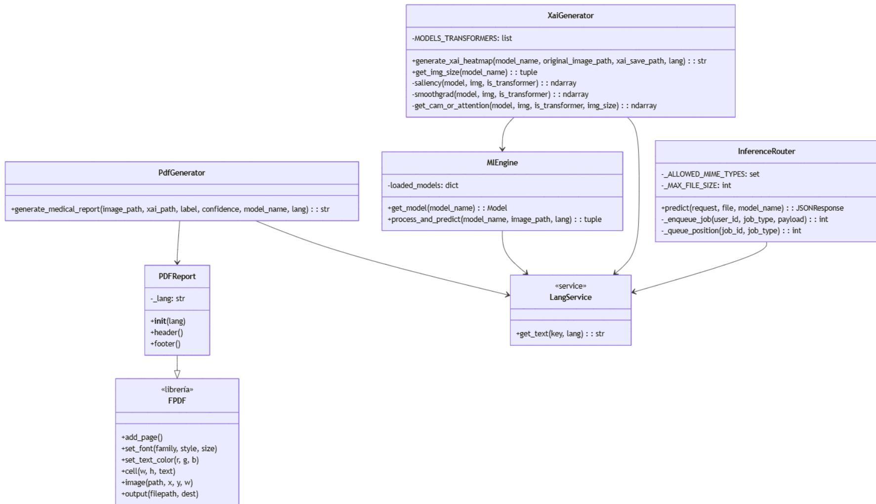
Ilustración 71 - Diagrama de clases del subsistema SD-002
