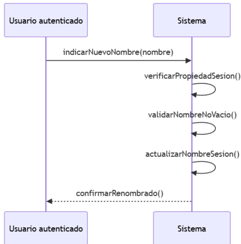
Ilustración 51 - Secuencia de interacción del renombrado de una sesión (CU-029)
