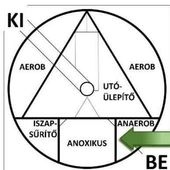
1. ábra: az oltóanyag bejuttatása az Anaerob kamrába
