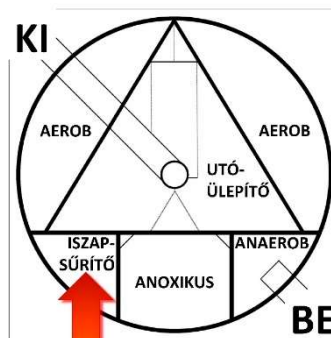
2. ábra: az Iszapsűrítő kamrába vezető iszapelvételi könyök
