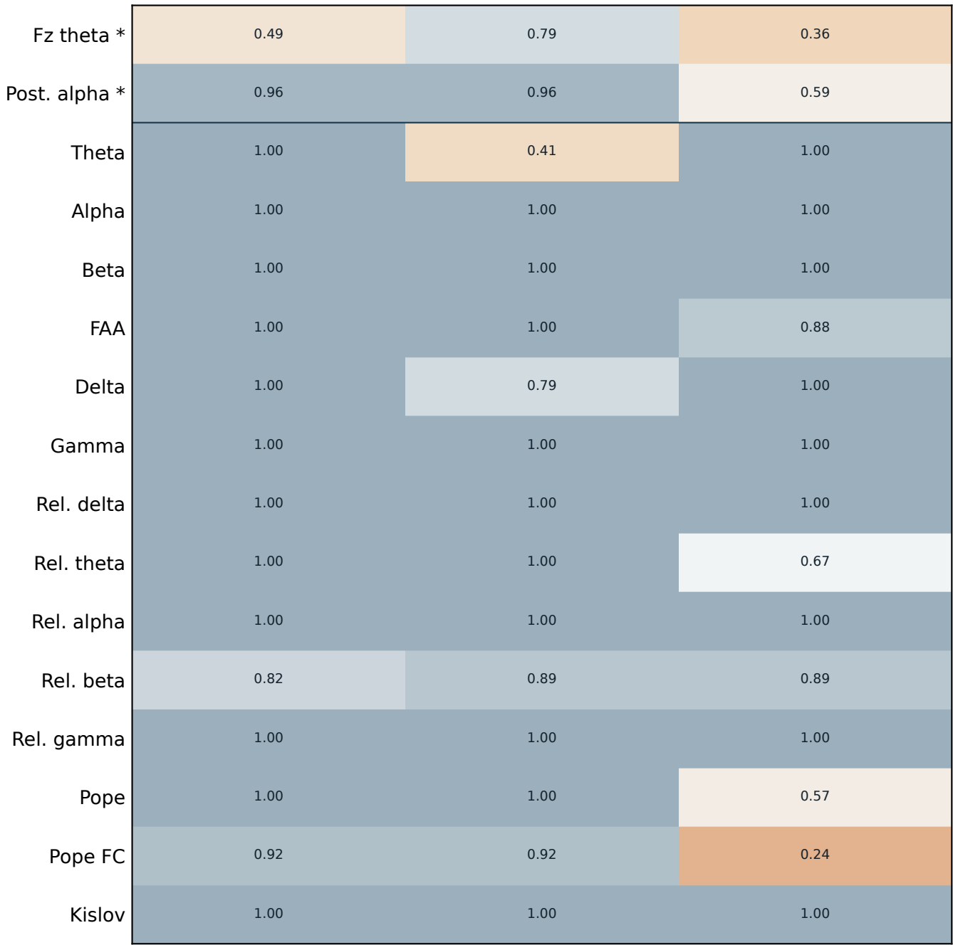
Dataset A Holm p · 4 s · ICA
