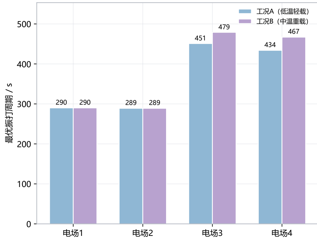
(b) 四级电场最优振打周期
