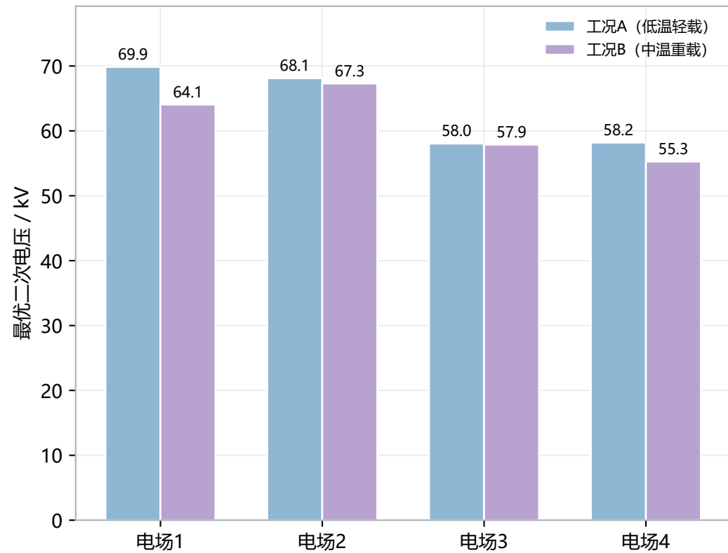
(a) 四级电场最优电压
