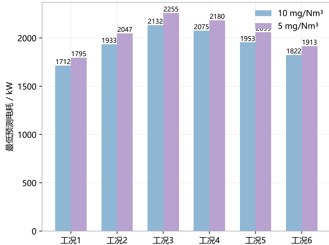
(a) 可行工况最低电耗
