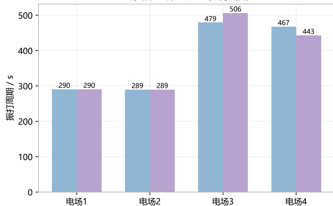
高负荷重载工况5：振打周期
