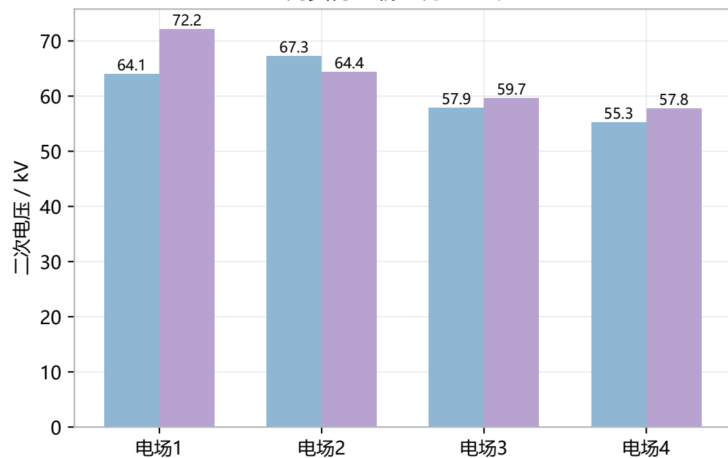
高负荷重载工况5：电压
