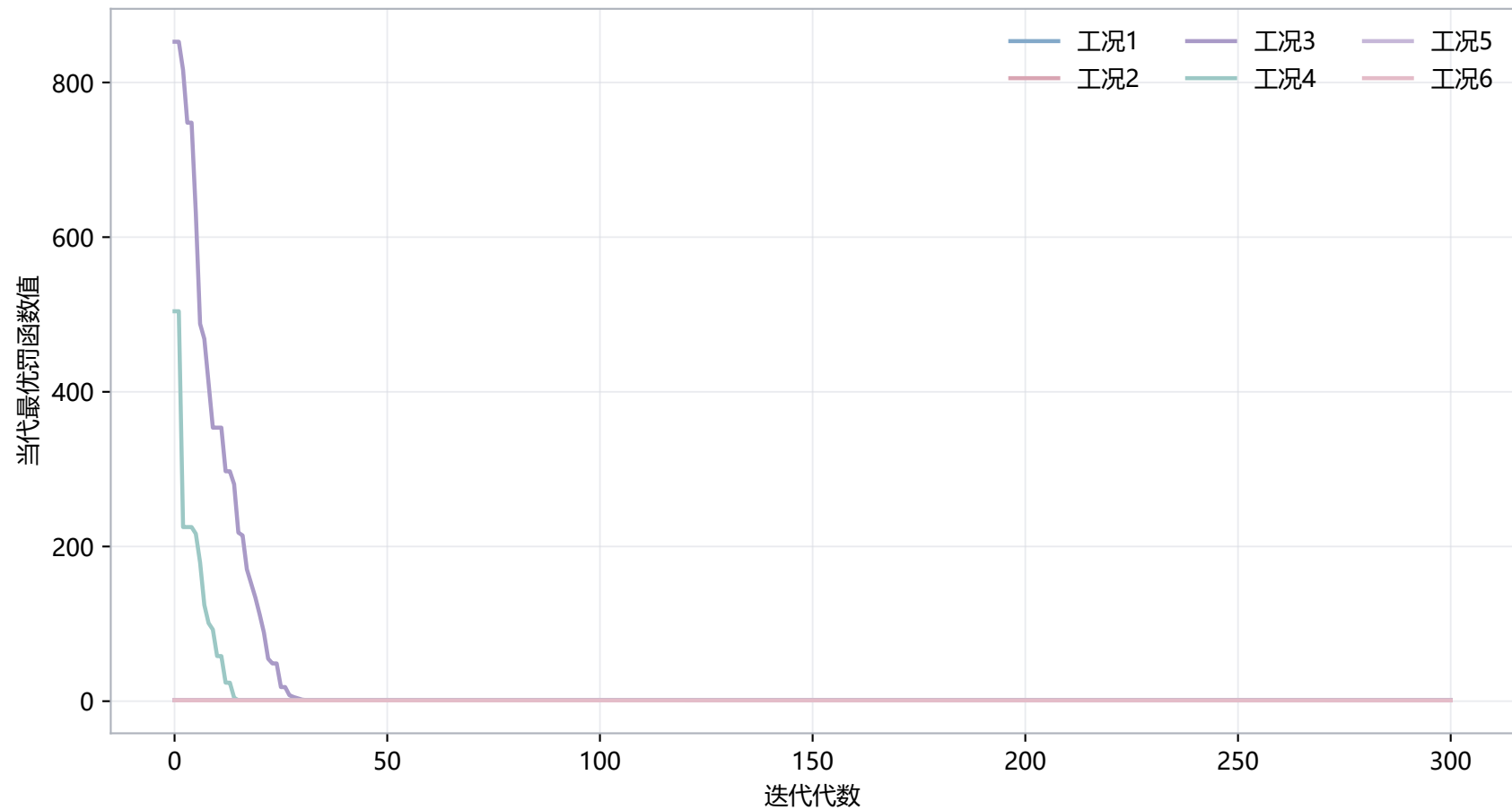
遗传算法罚函数收敛过程
