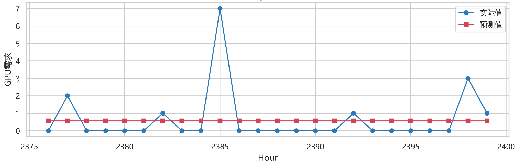
SBA-Croston示例: RegionF - RealTimeInference
