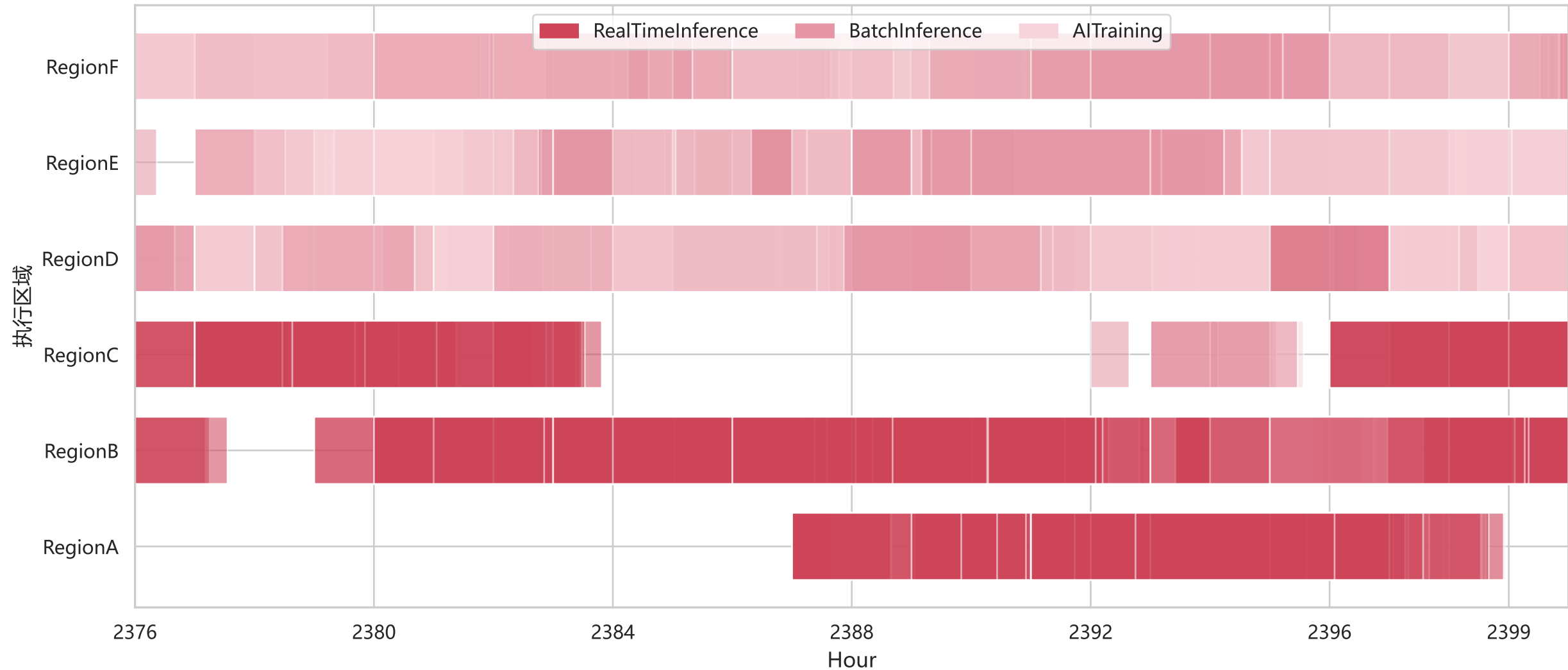
2376—2399时段任务调度甘特图
