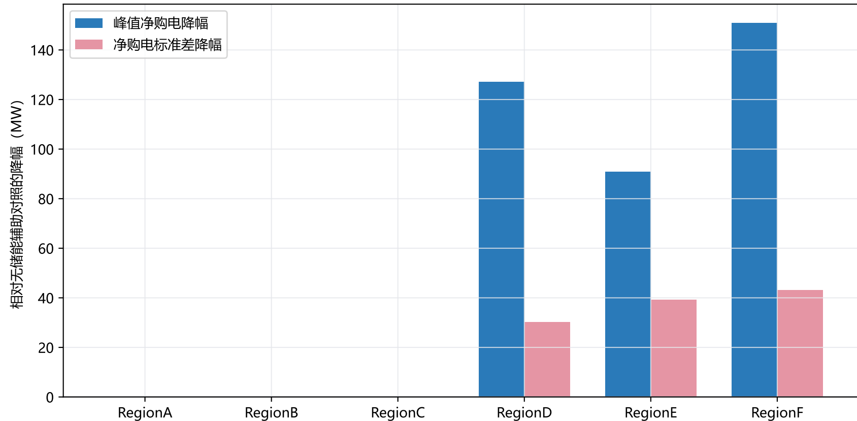
等权储能方案的区域峰值与波动增量影响
