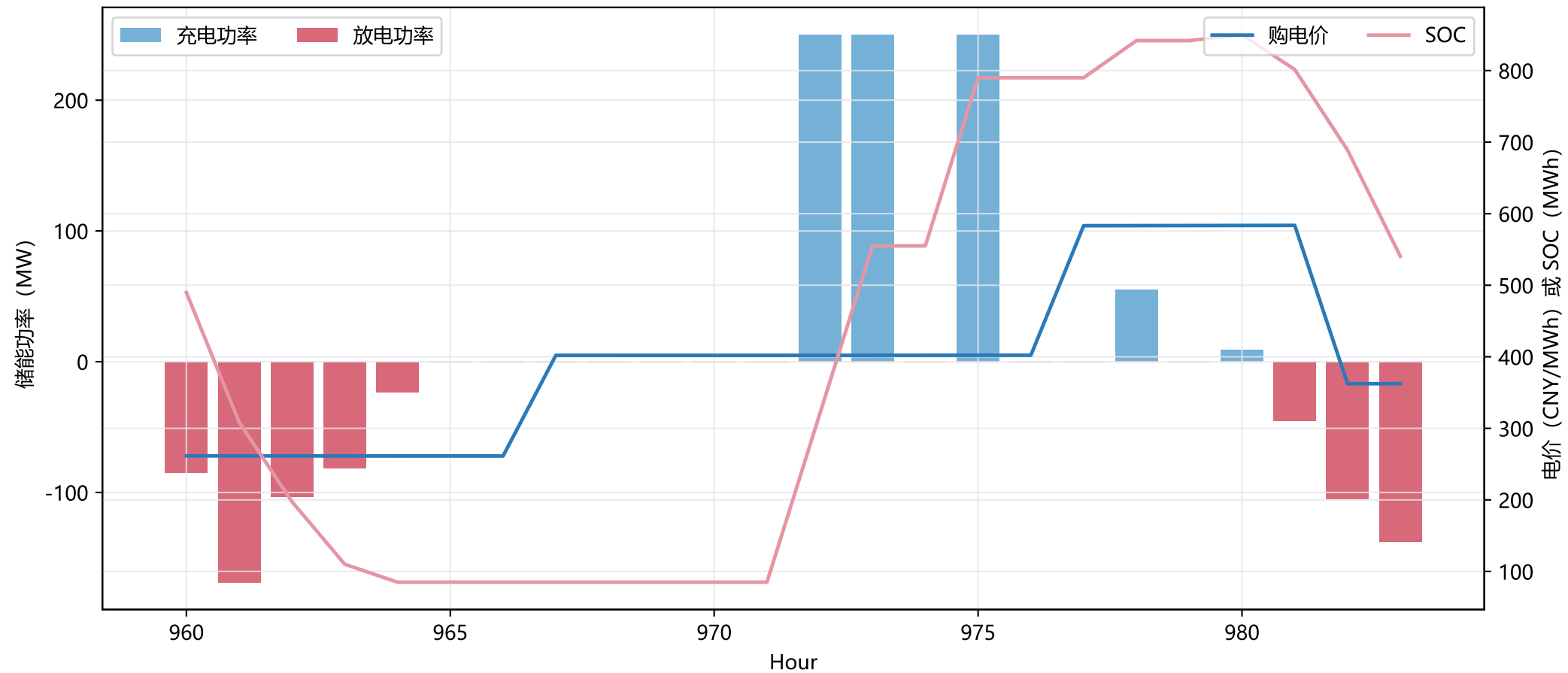
RegionF 第40日储能运行轨迹
