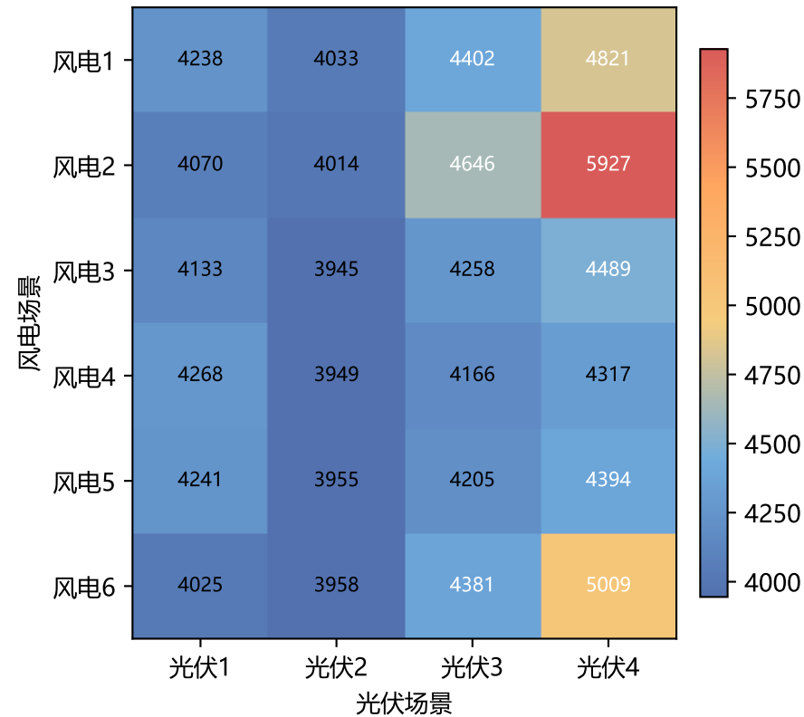
净吨氨成本 / ¥/t
