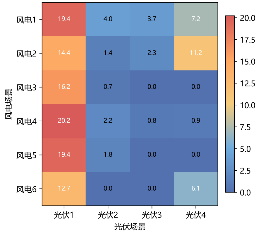
弃电率 / %
