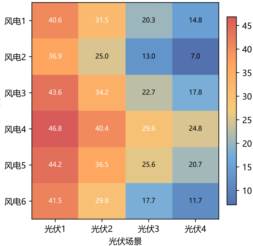
日氨产量 / t/day
