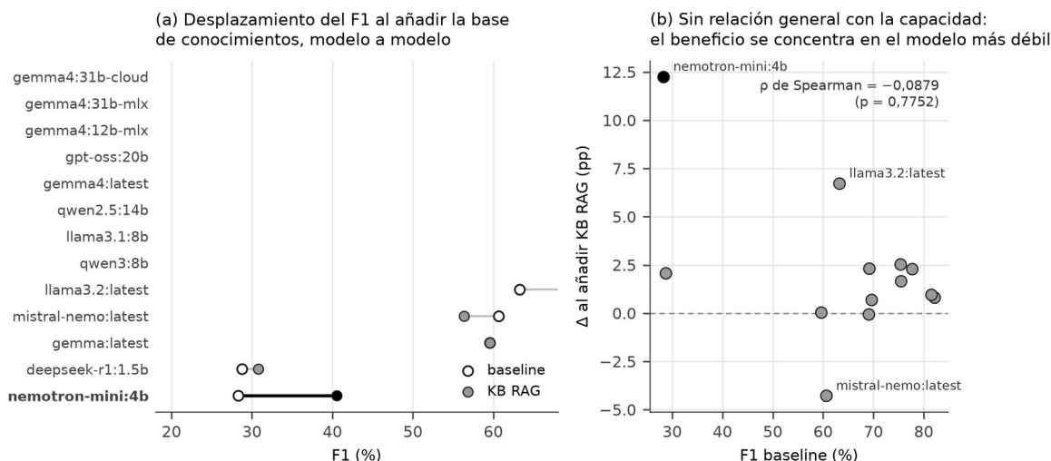
Figura 1. Efecto de la base de conocimientos contextual sobre los trece modelos (N=120). El panel (a) une con un trazo el F1 de cada modelo sin recuperación y con ella; en negro, el único caso en que la mejora supera la corrección por comparaciones múltiples. El panel (b) representa esa misma mejora frente al desempeño de partida. Elaboración propia a partir de la Tabla 7
