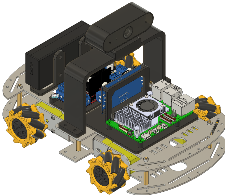
หุ่นยนต์ต้นแบบ Raspberry Pi 4 ล้อ Mecanum 4 ล้อ กล้องด้านบน
