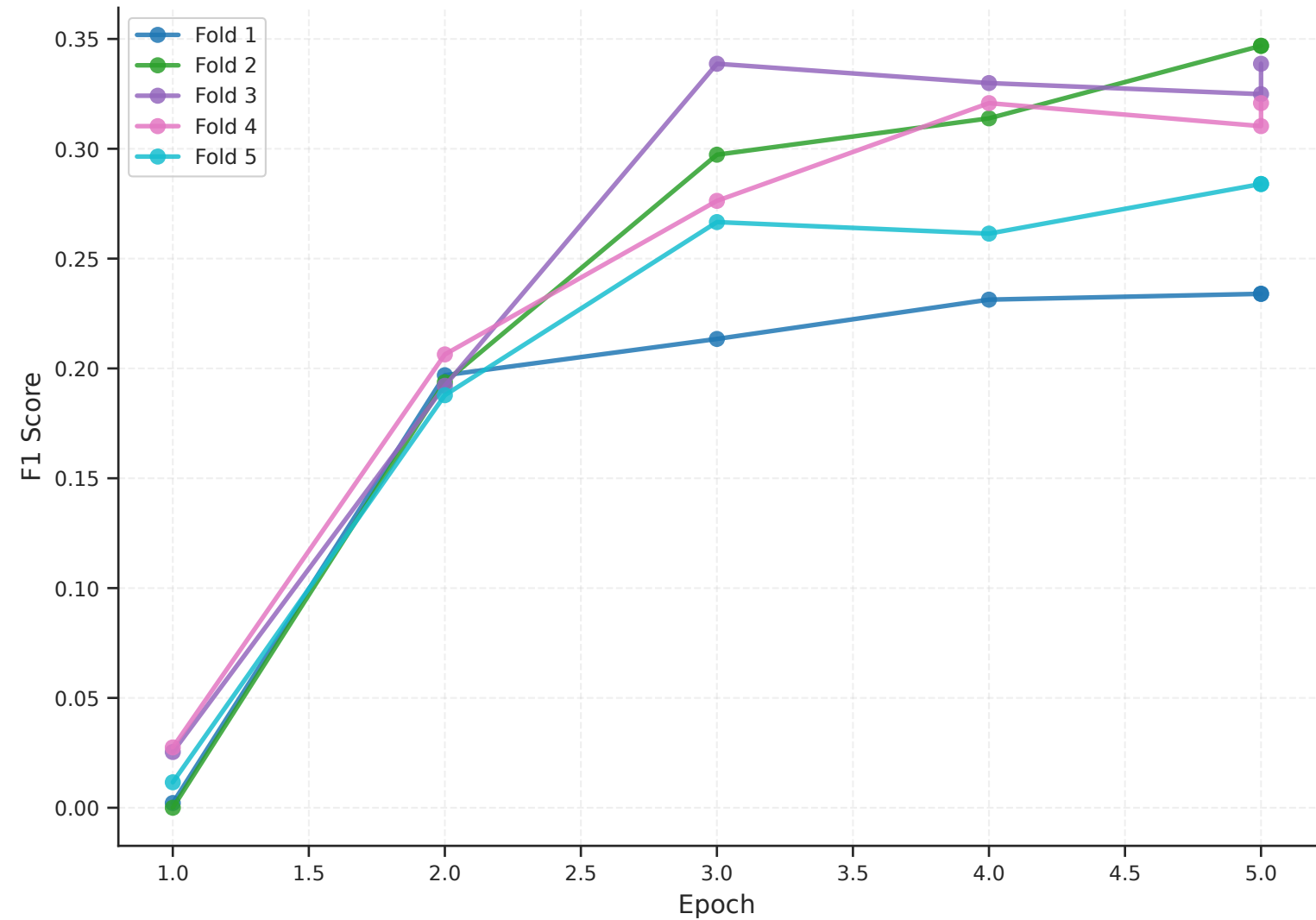
F1 Macro Score - twitter-roberta-base-hate-multiclass-latest
