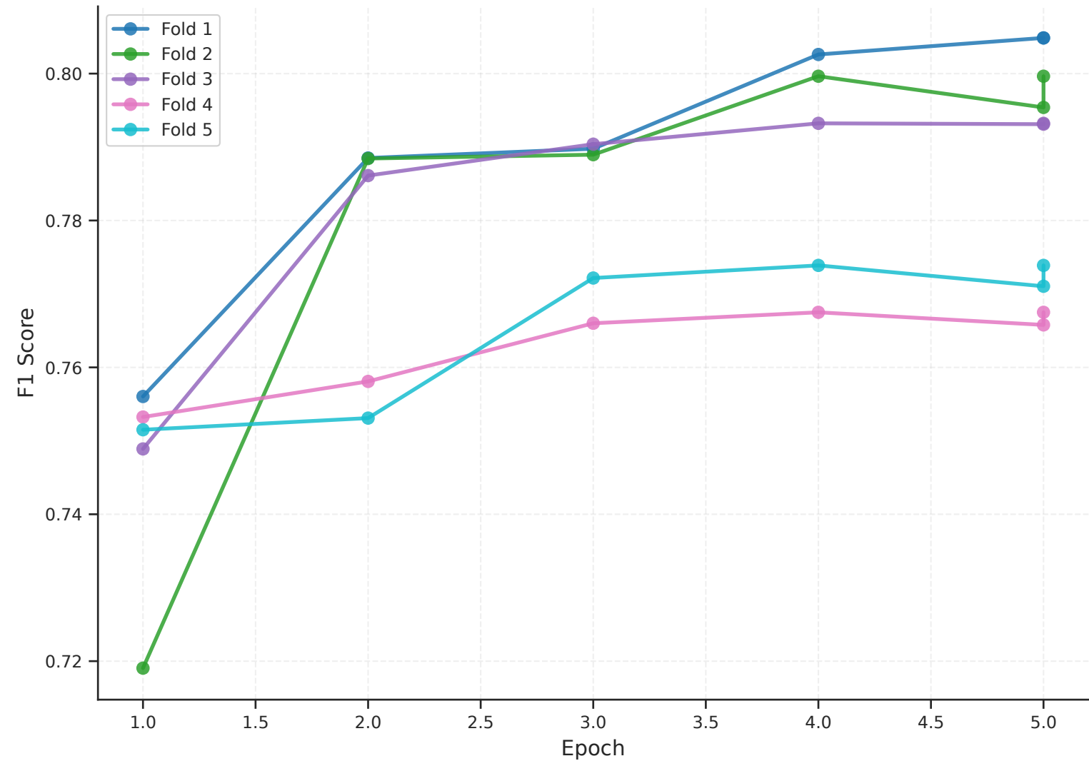
F1 Macro Score - afro-xlmr-base
