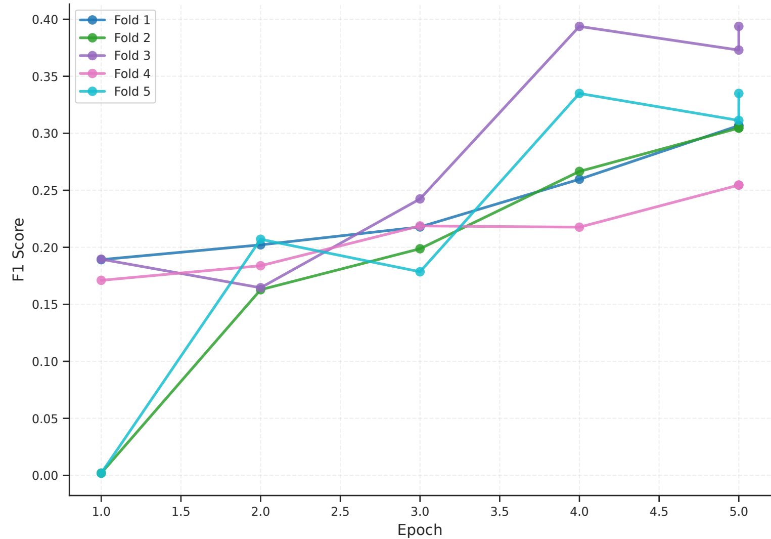
F1 Macro Score - deberta-v3-base
