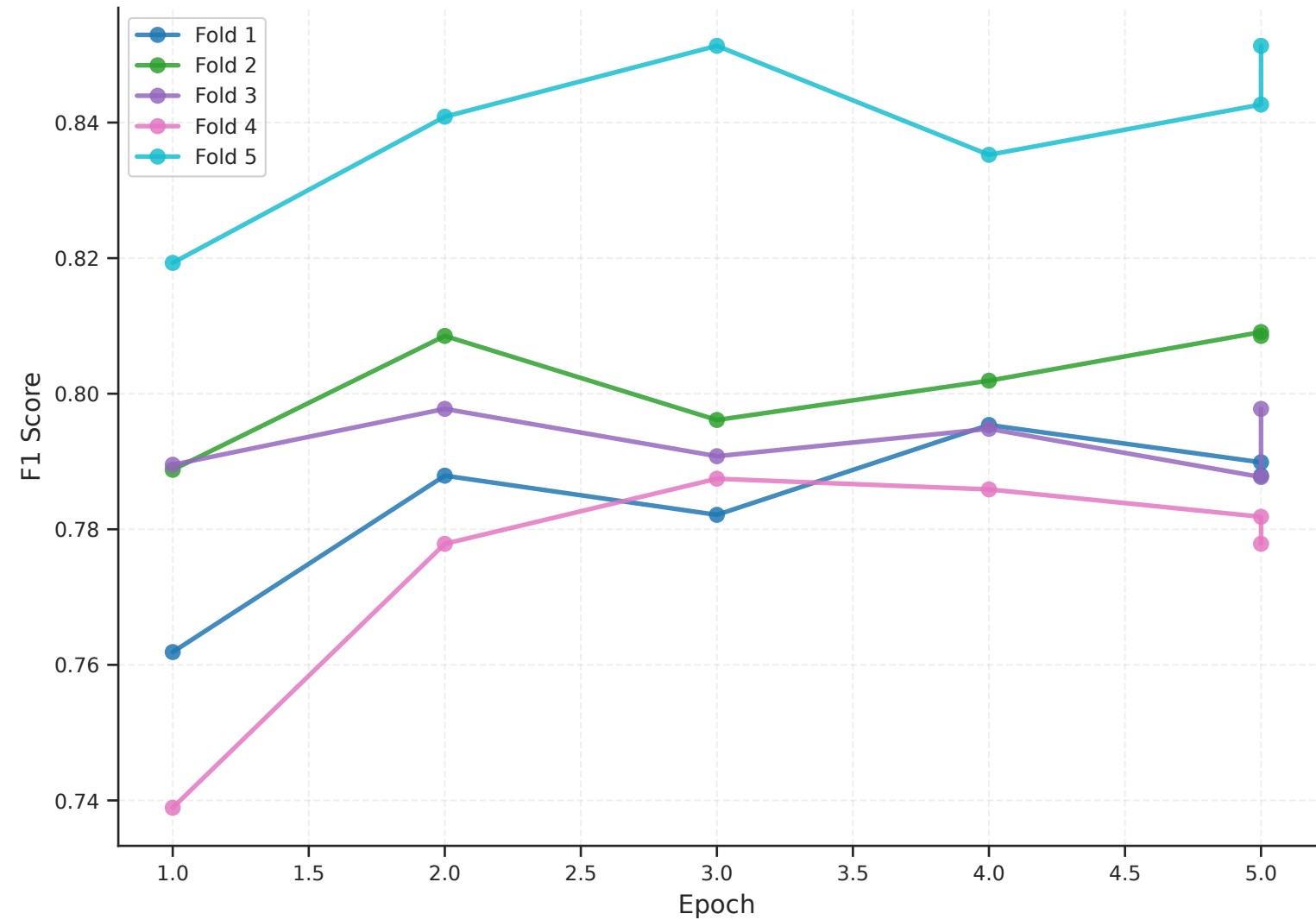
F1 Macro Score - twitter-roberta-base-hate-latest
