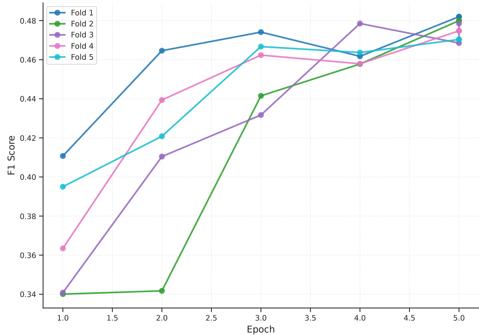
F1 Macro Score - swahBERT
