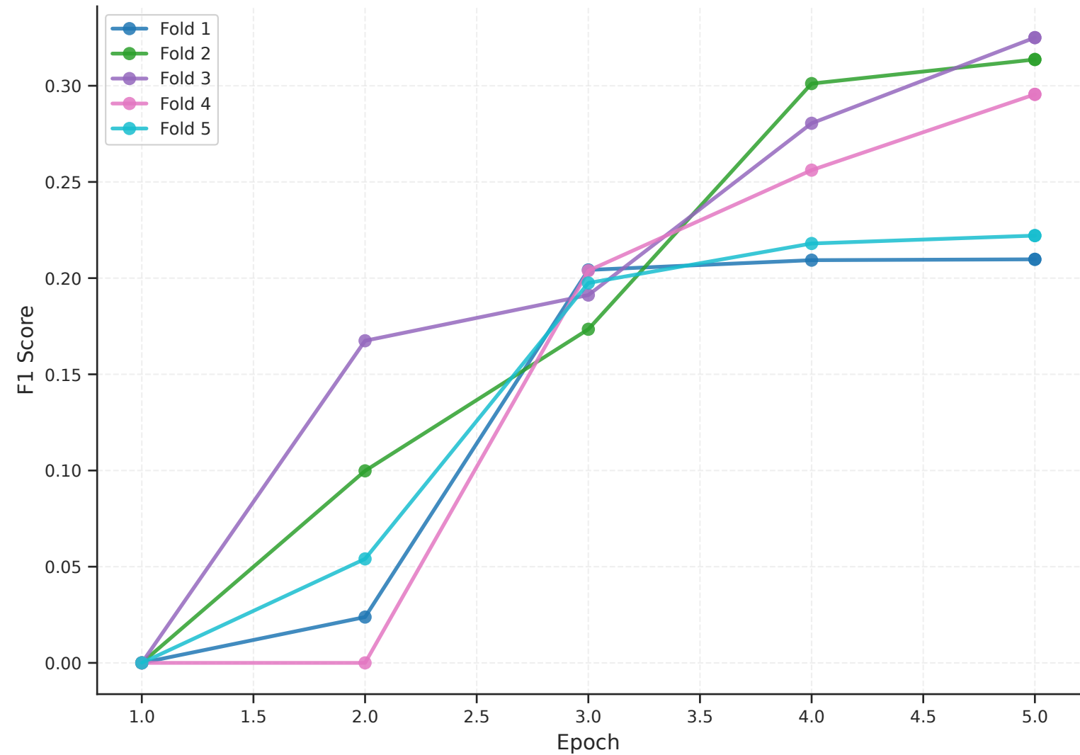
F1 Macro Score - twitter-roberta-base-2022-154m
