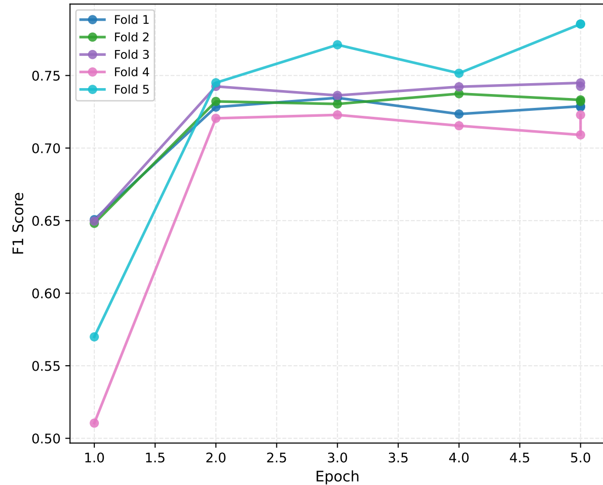
F1 Macro Score - All Folds
