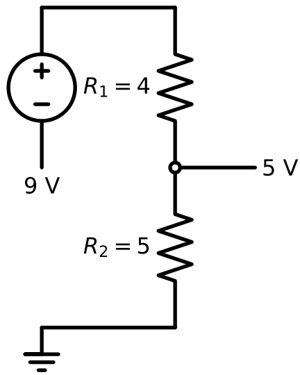
Figura 1: Divisor de tensión
