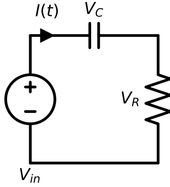
Figura 1: Circuito RC
