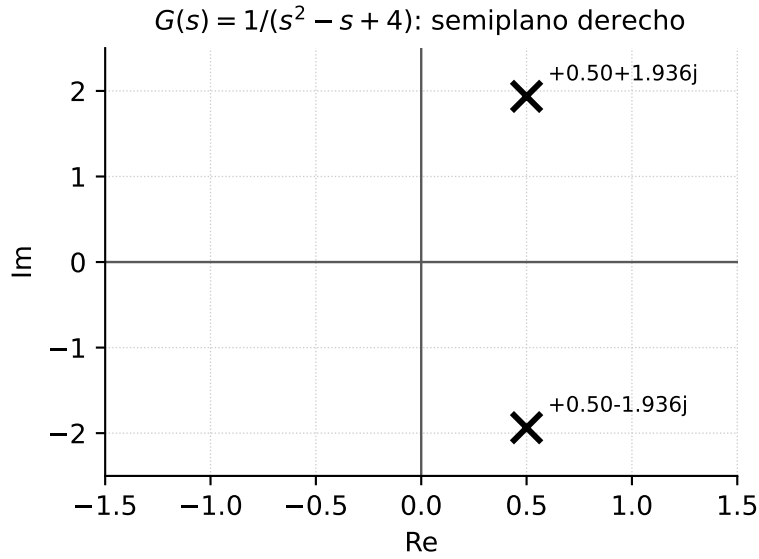
Figura 2.3: Polos en el semiplano derecho
