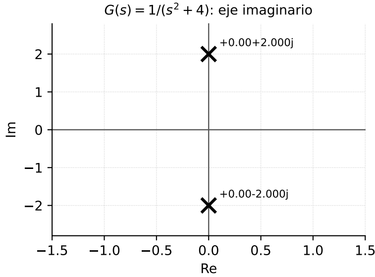
Figura 2.4: Polos sobre el eje imaginario
