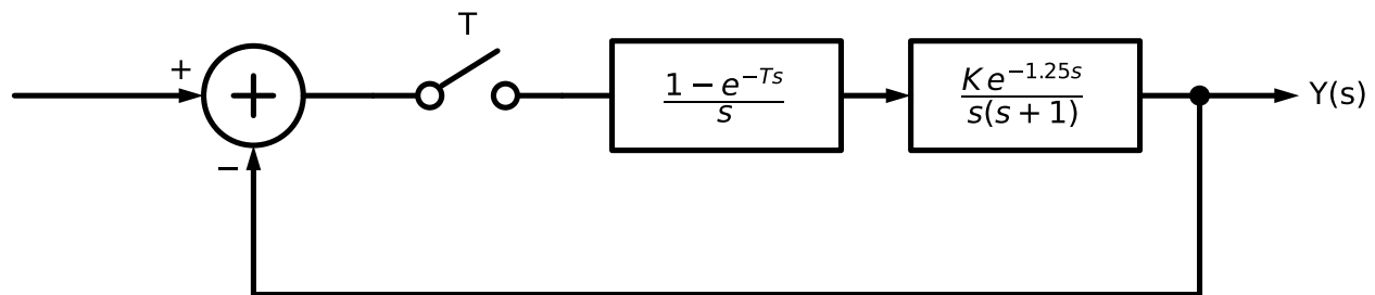
Figura 4.2: Lazo muestreado con ZOH
