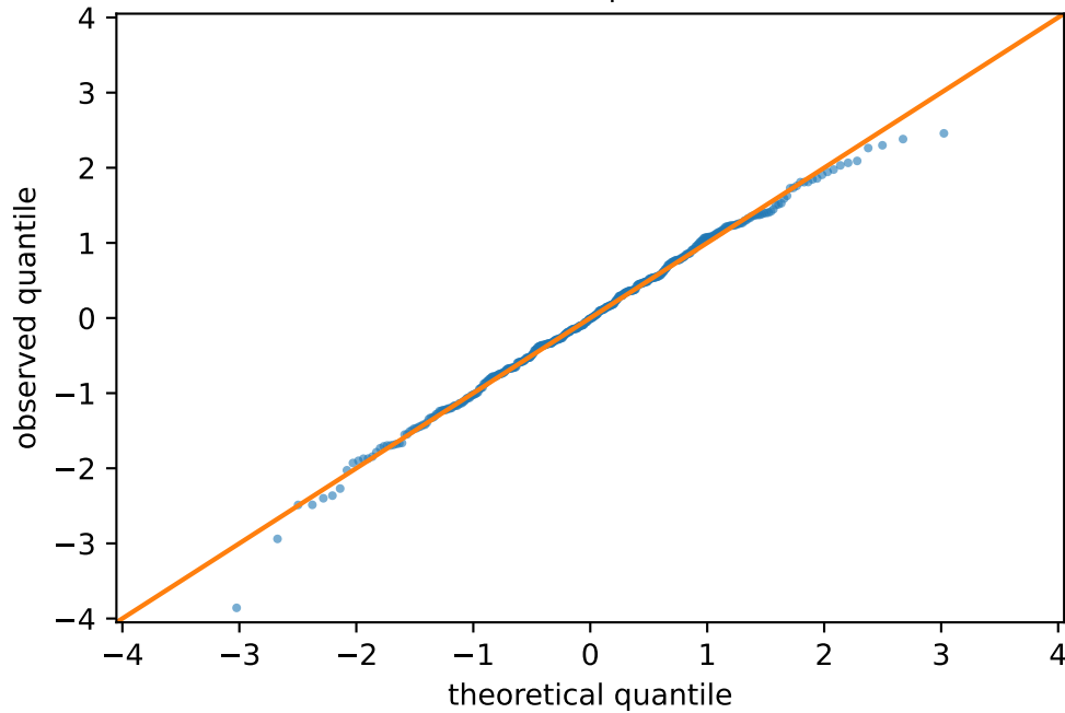
Quantile-quantile
