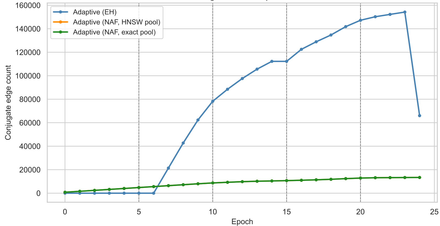
Edge Count vs Epoch
