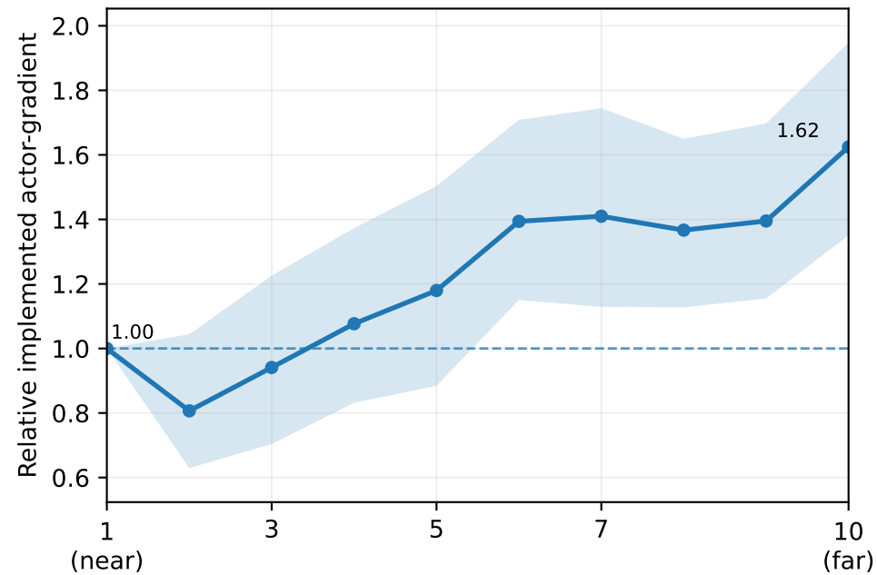
mini sudoku near->far = 1.62x
