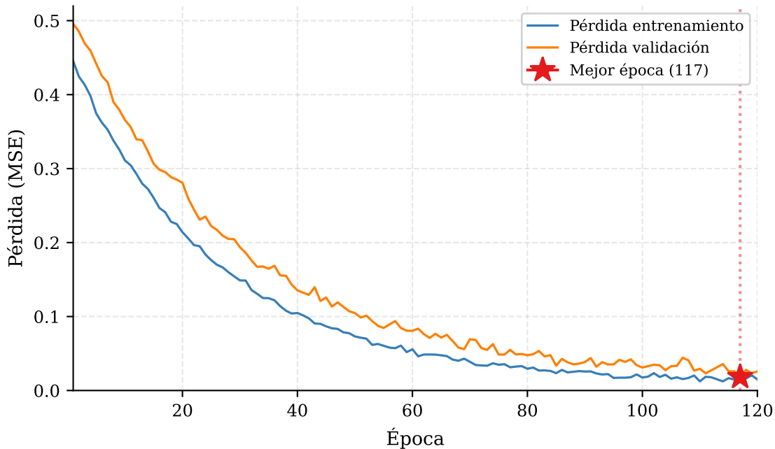
Fig. 3 – Convergencia del entrenamiento (LSTM propuesto)
