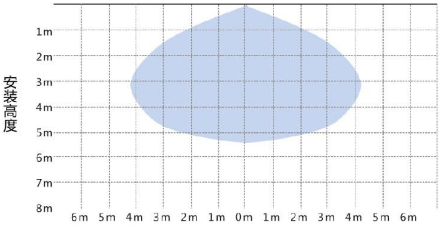
雷达感应示意图
