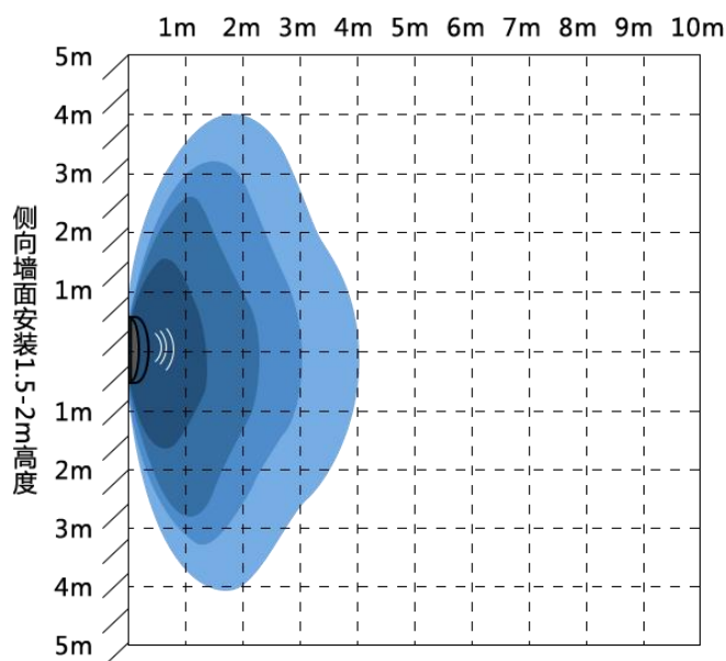
壁挂式安装图
