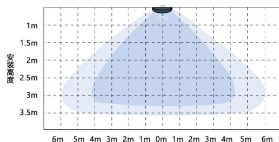
吸顶安装图
