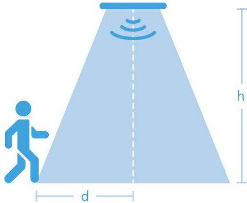
挂高 3m，感应距离为 3-4m（半径）
