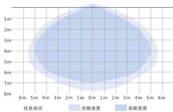
吸顶安装图
