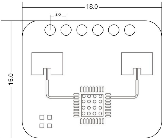
EDQ182 (尺寸公差 10%) 板厚 1.6mm 单位： (mm)
