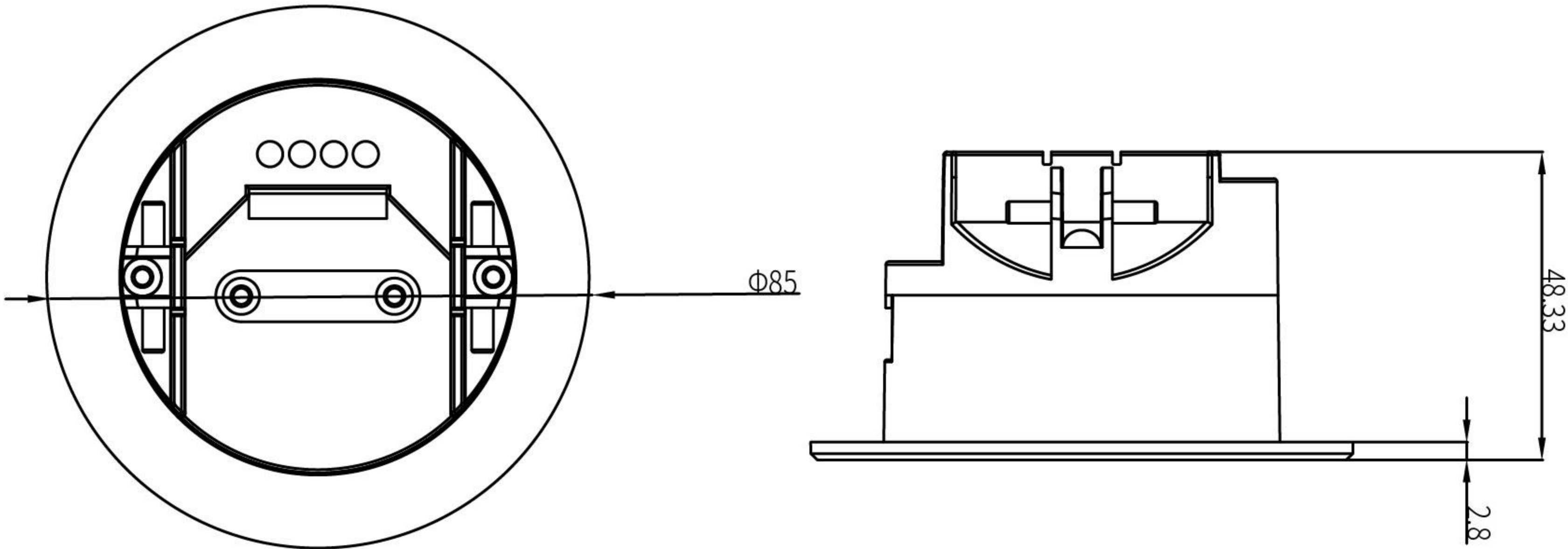
EDQ282 尺寸公差: ±0.2
