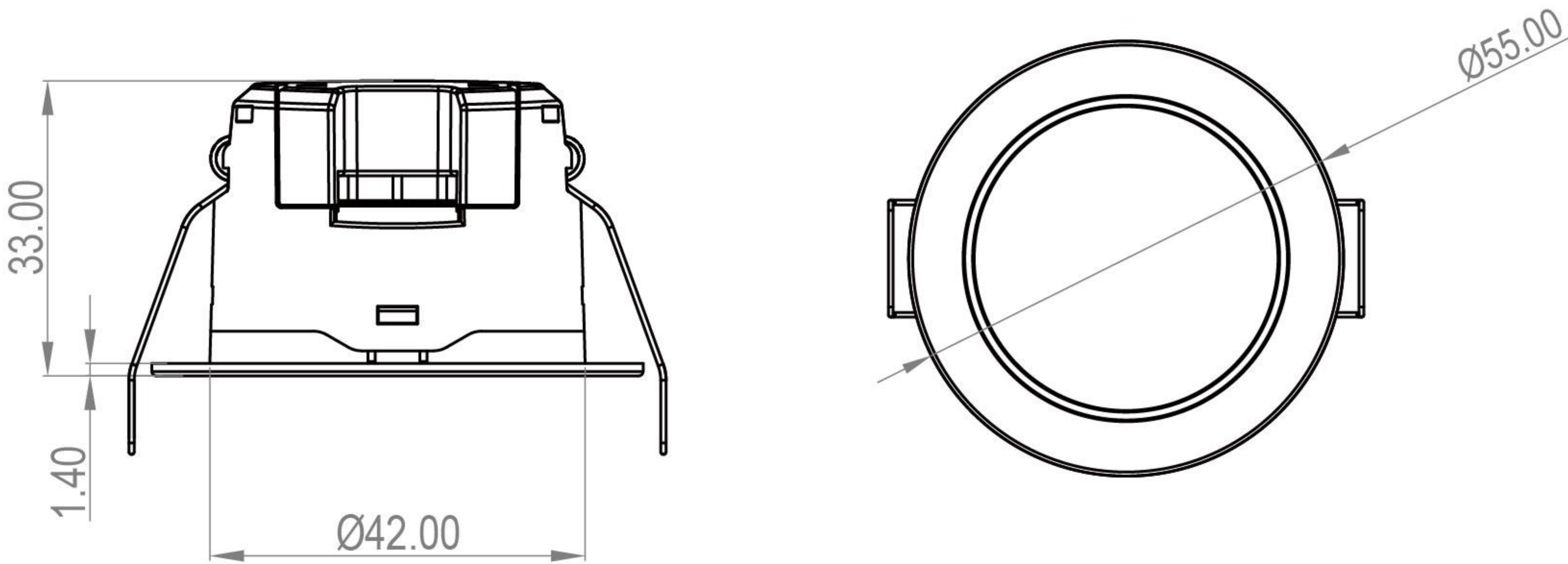
EDQ286 尺寸公差: ±0.2mm
