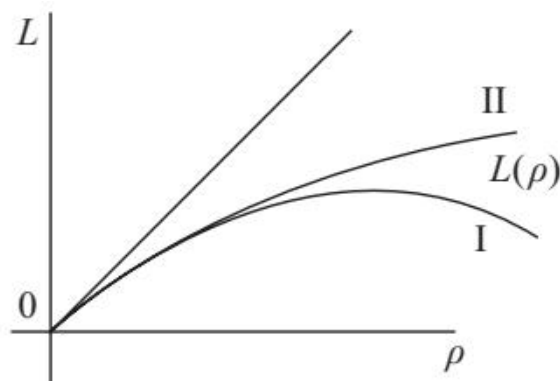
(b) K > 0 : 测地线先远离后靠近
