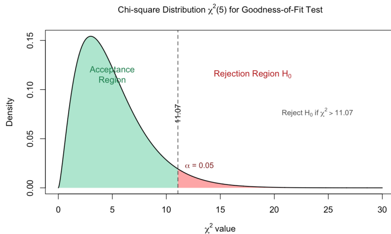
图 2. 自由度为 5 的卡方分布，显著性水平 \alpha = 0.05 的拒绝域（右侧尾部）。当检验统计量 \chi^2 > 11.07 时，拒绝原假设。
