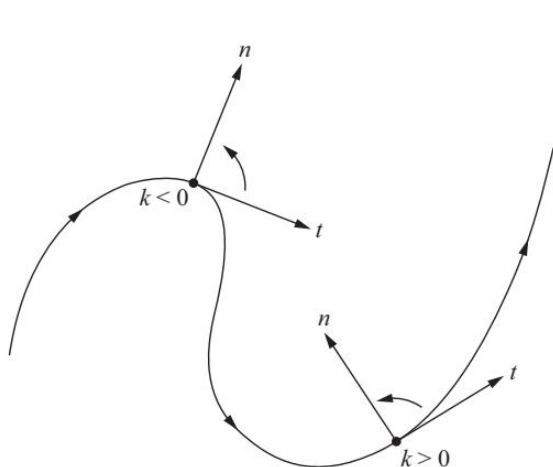
(a) Figure 1-16 (a). 有向曲率 - 正向
