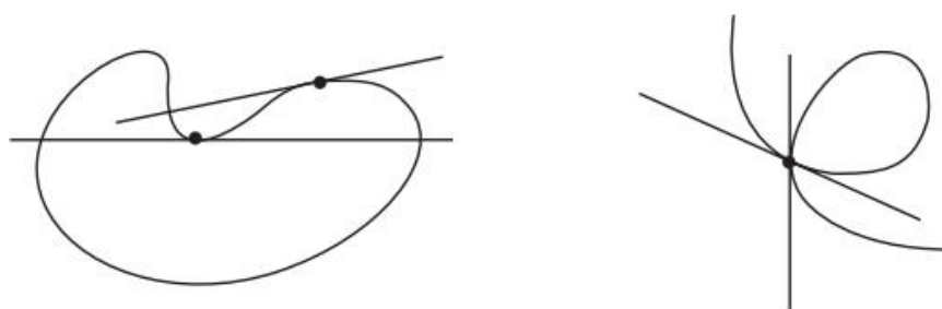
(a) Figure 1-28 (b). 非凸曲线
