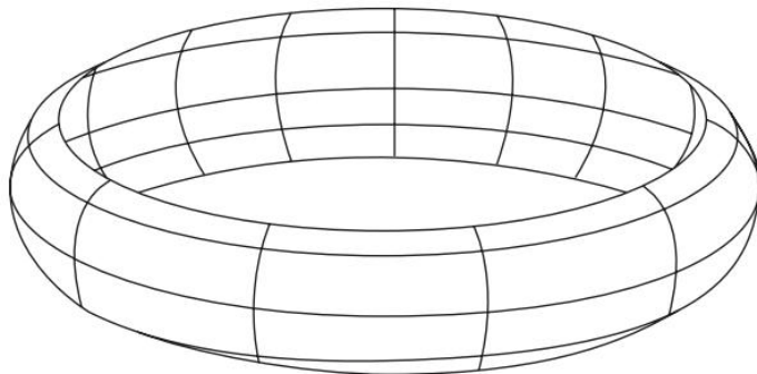
(a) Figure 5-2. 常正曲率旋转面
