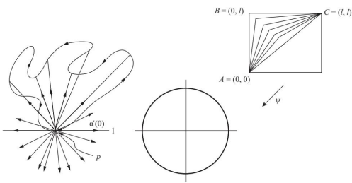
(a) Figure 5-33. 旋转定理的证明：割线映射
