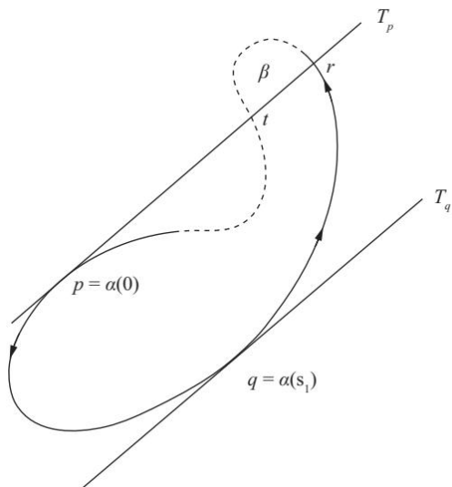
(a) Figure 5-42. Stoker 定理证明中的自交构造
