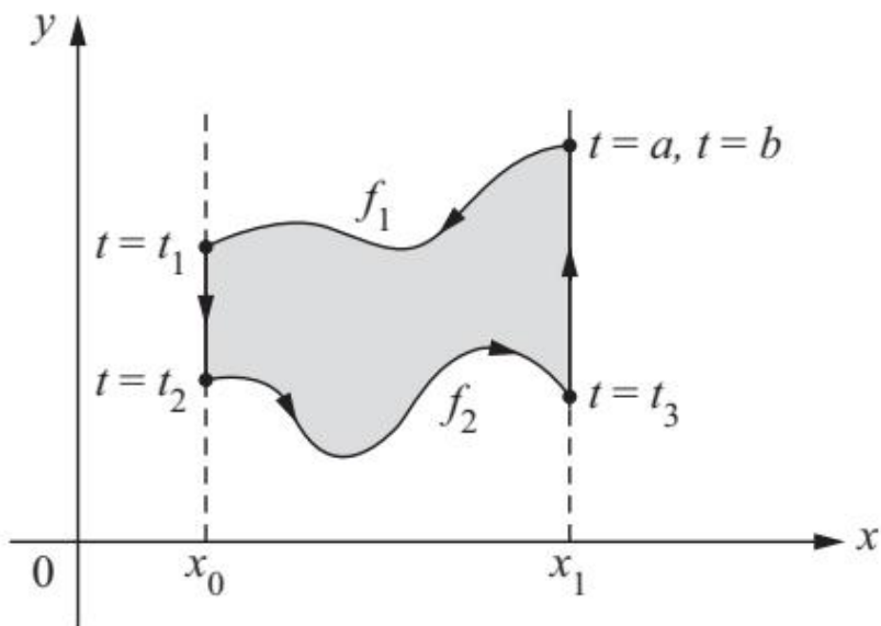
(a) Figure 1-22. 等周公式证明图示
