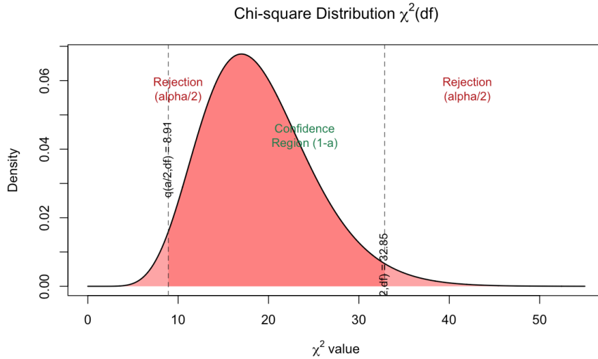
图 1. \chi^2 分布的置信区间示意图。图中阴影区域为置信区间 [(n-1)S^2/\chi^2_{\alpha/2, n-1}, (n-1)S^2/\chi^2_{1-\alpha/2, n-1}] 对应的统计量 (n-1)S^2/\sigma^2 的取值范围，两侧红色区域为显著性水平 \alpha/2 的拒绝域。
