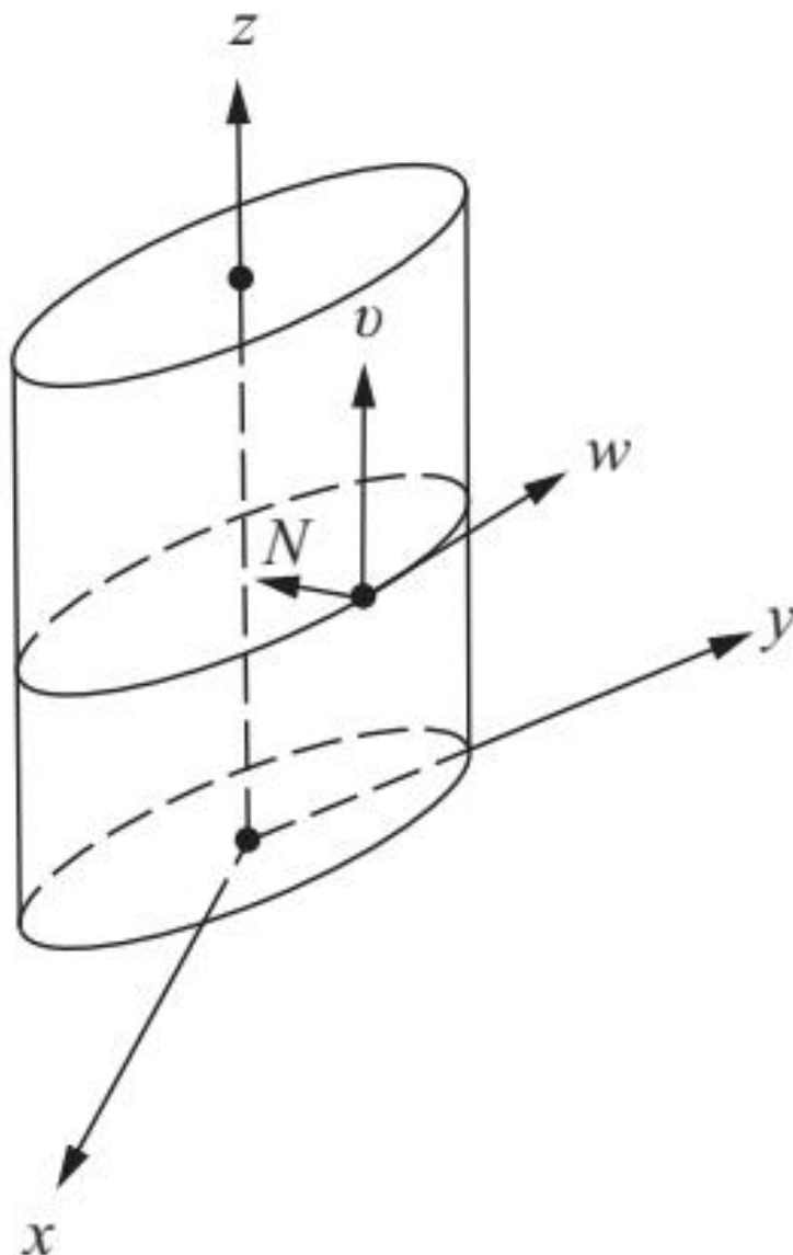
(a) Figure 3-6. 圆柱面的 dN
