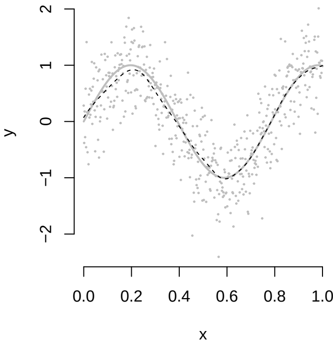
local linear fit
