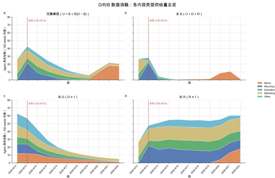
图 4 B、D、R 单因素消融下的 Agent 供给构成。
