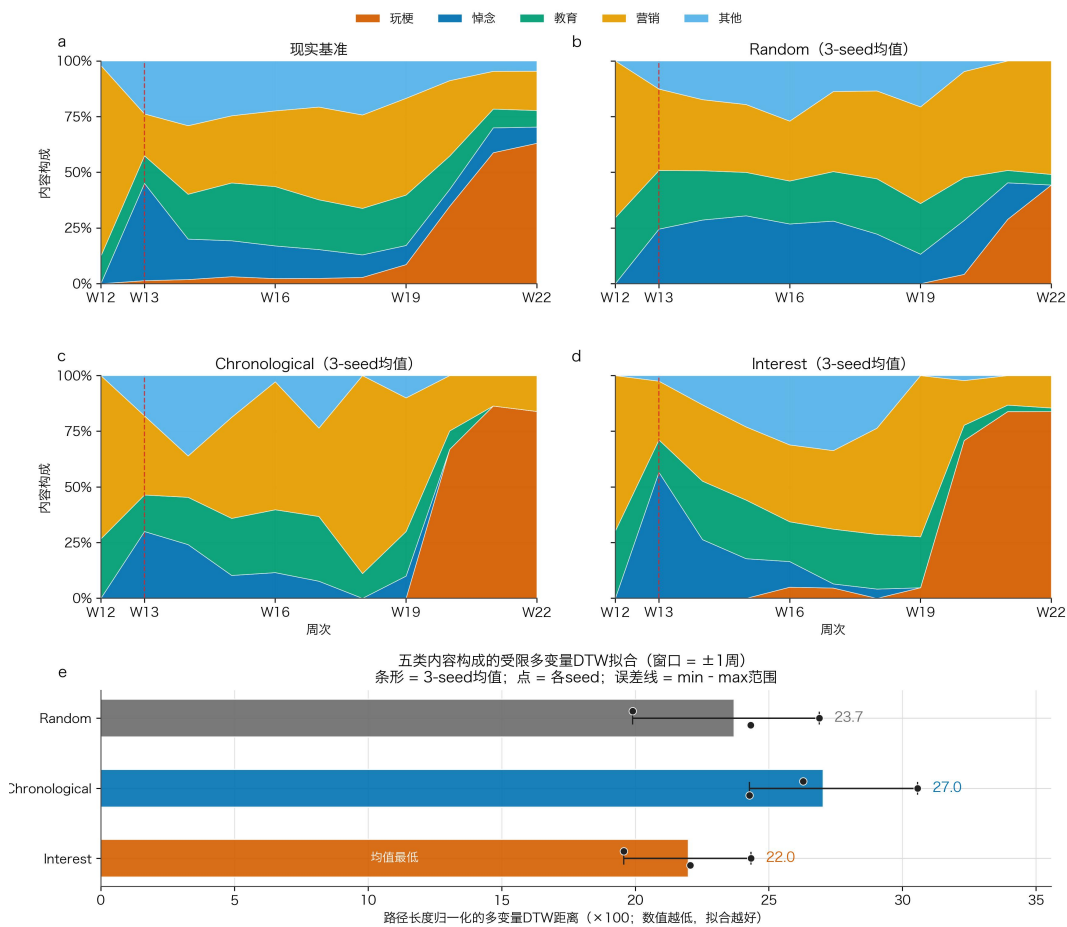
图2 五类表征轨迹的现实复现与受限多变量 DTW 拟合
