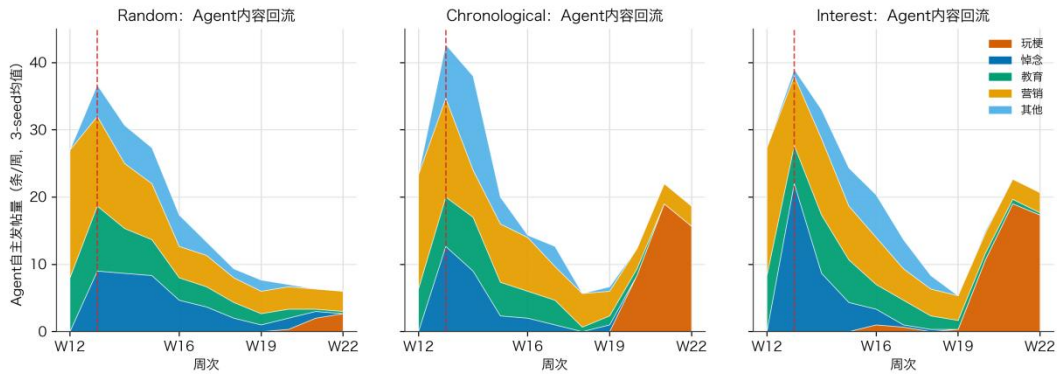
图 3b 三种策展制度下的 Agent 内容回流
