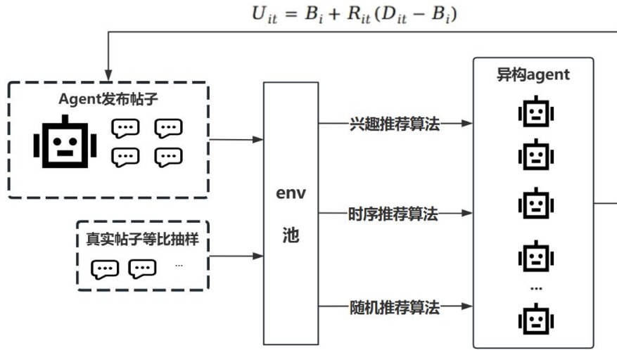
图1 多智能体模拟构架图
