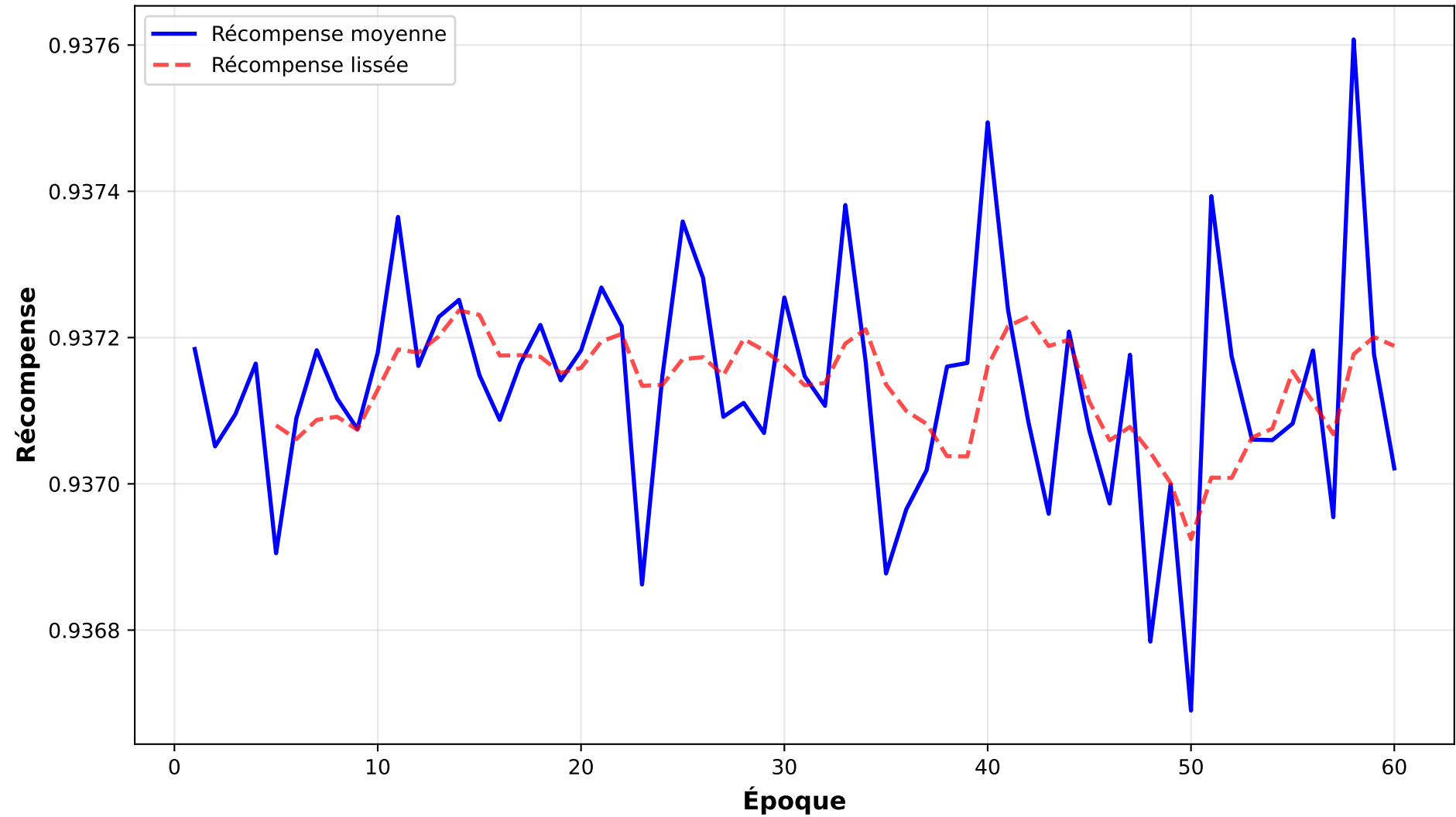
Courbe d'apprentissage - D-DSN-tvsum-split0
