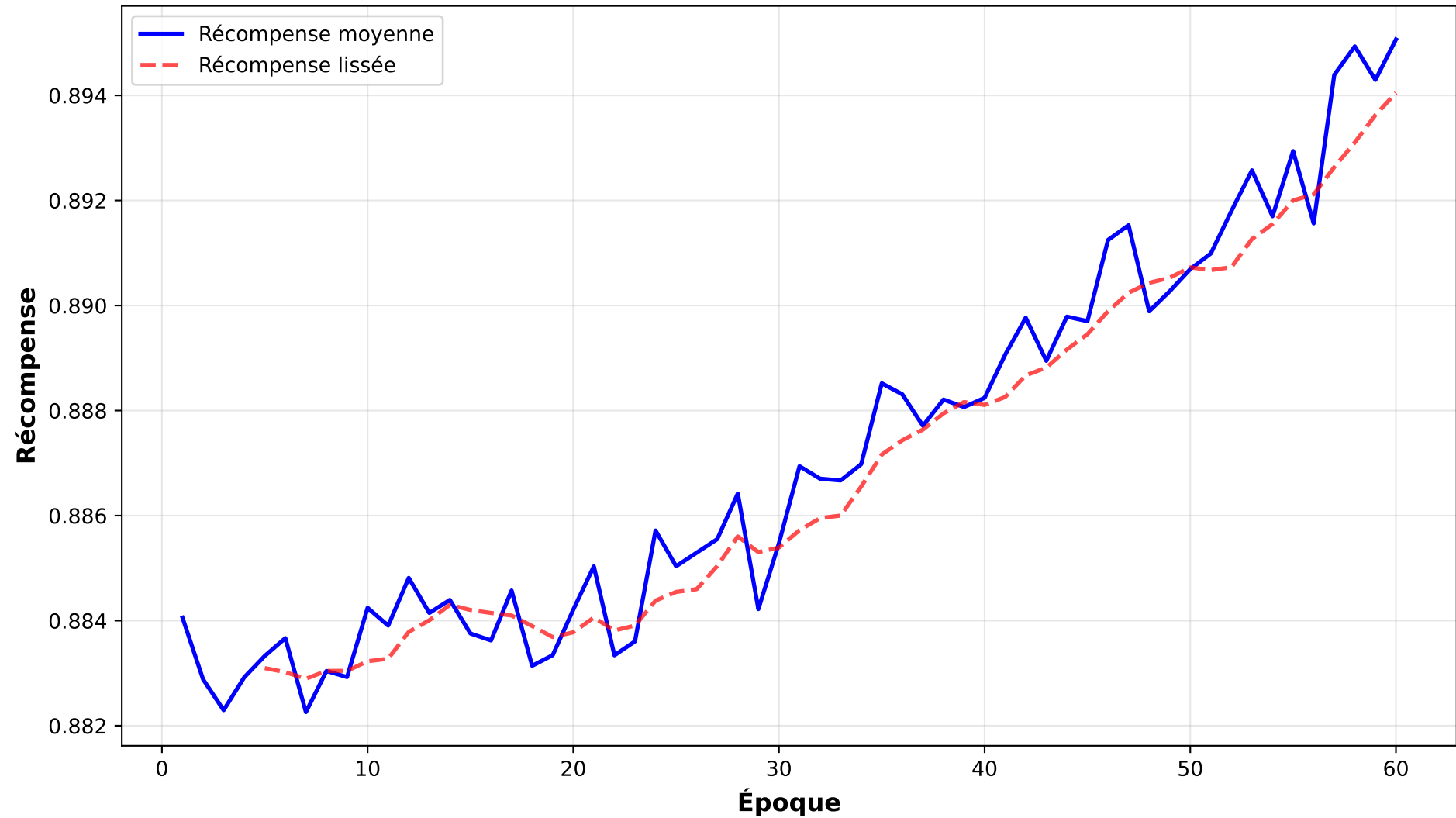
Courbe d'apprentissage - R-DSN-tvsum-split2
