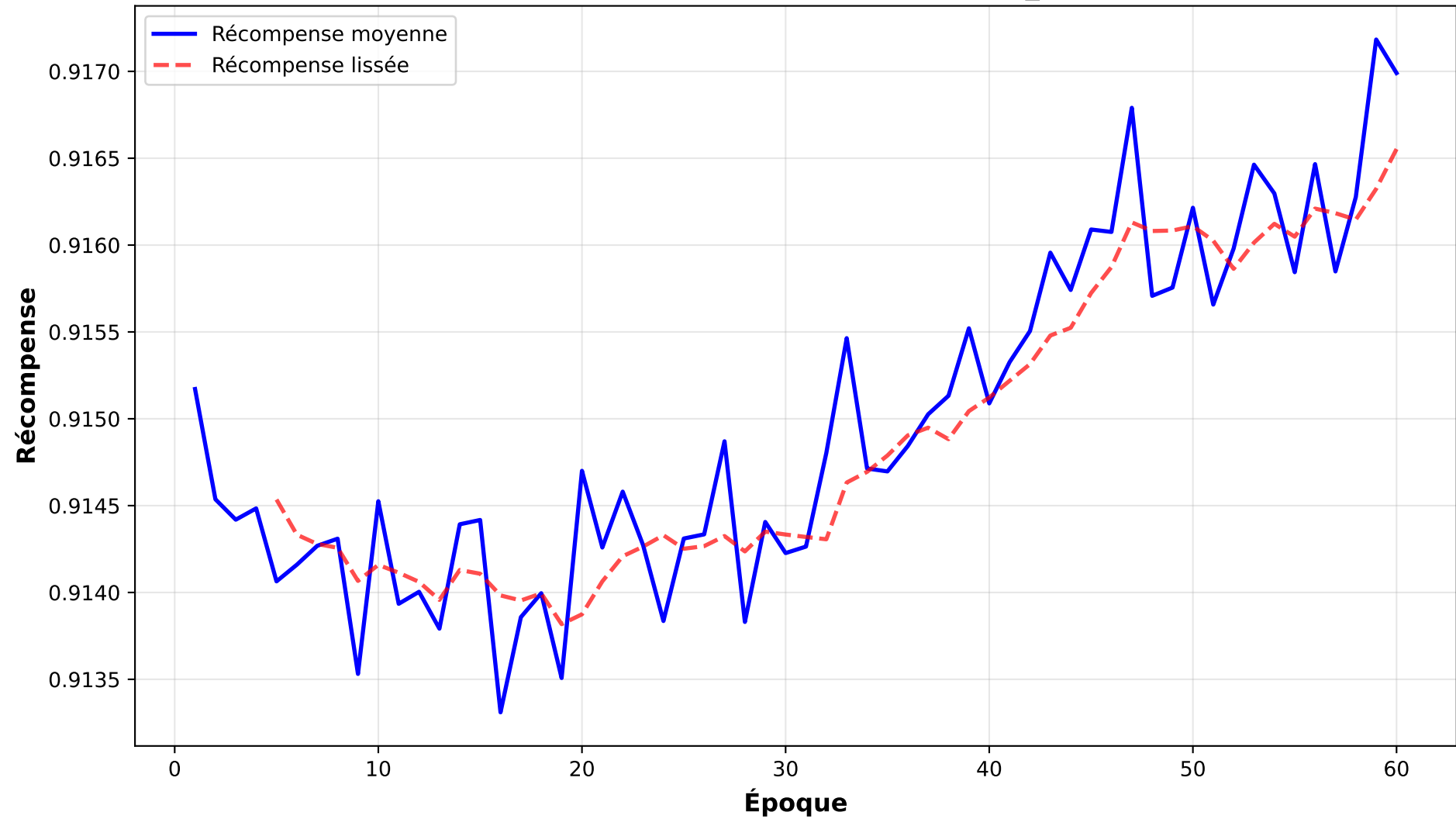
Courbe d'apprentissage - split_4
