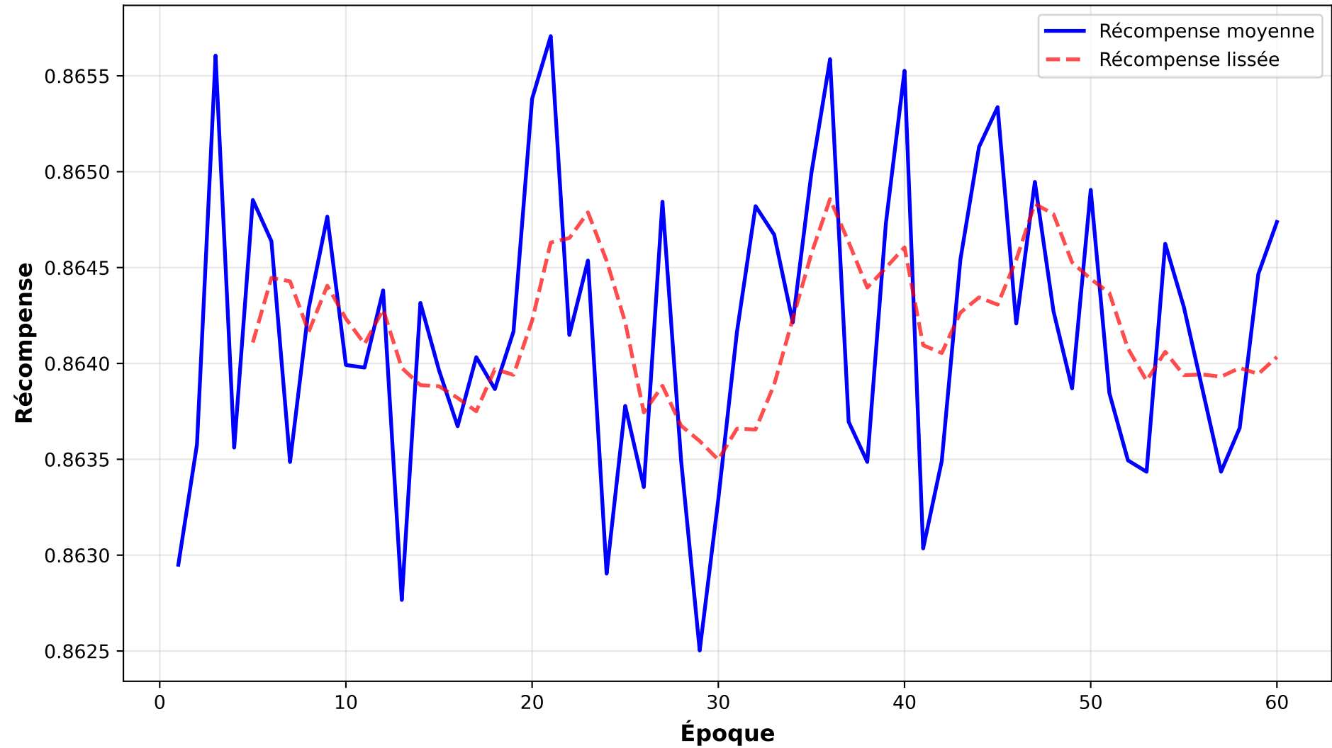
Courbe d'apprentissage - D-DSN-summe-split4
