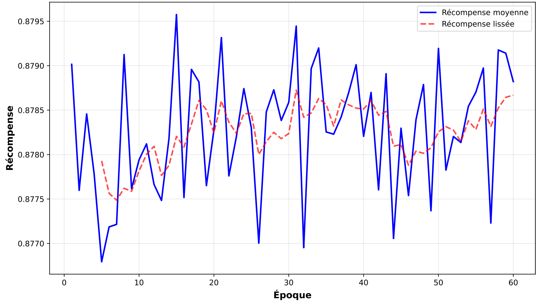
Courbe d'apprentissage - D-DSN-summe-split3
