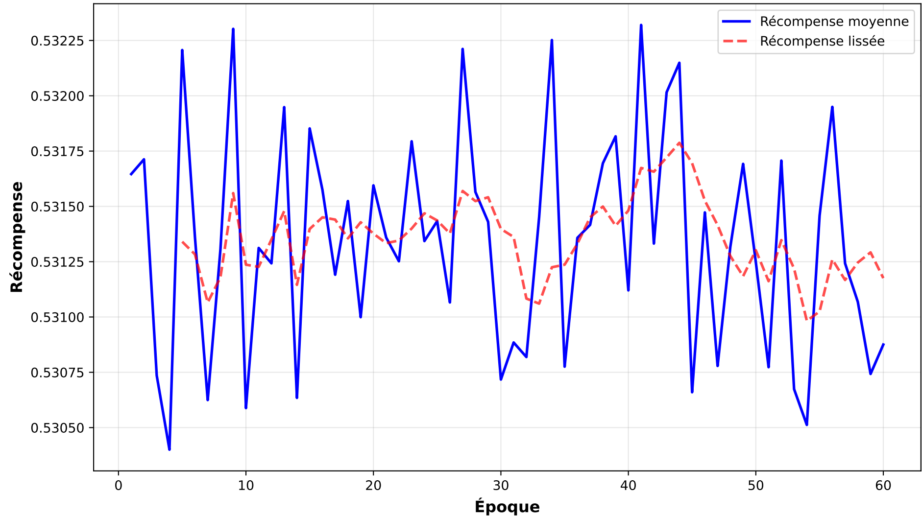
Courbe d'apprentissage - d-nolambda-tvsum-split3
