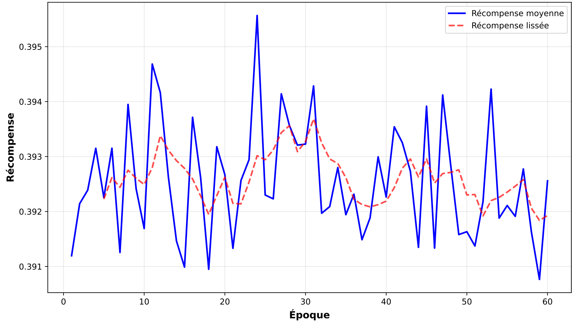
Courbe d'apprentissage - d-nolambda-summe-split2
