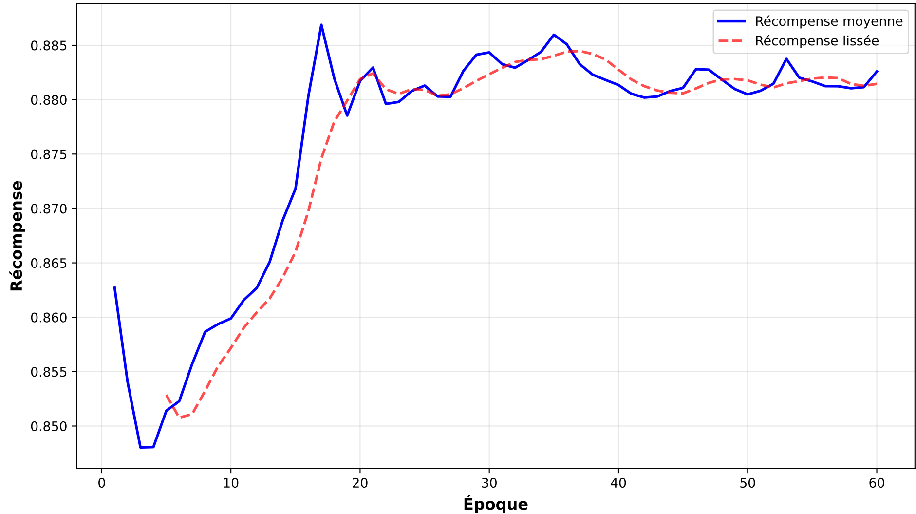
Courbe d'apprentissage - alt_run_dhash-optimized_split1
