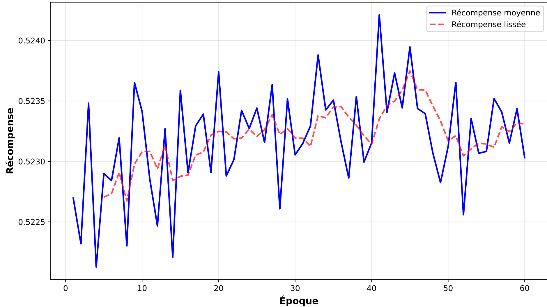
Courbe d'apprentissage - d-nolambda-tvsum-split2
