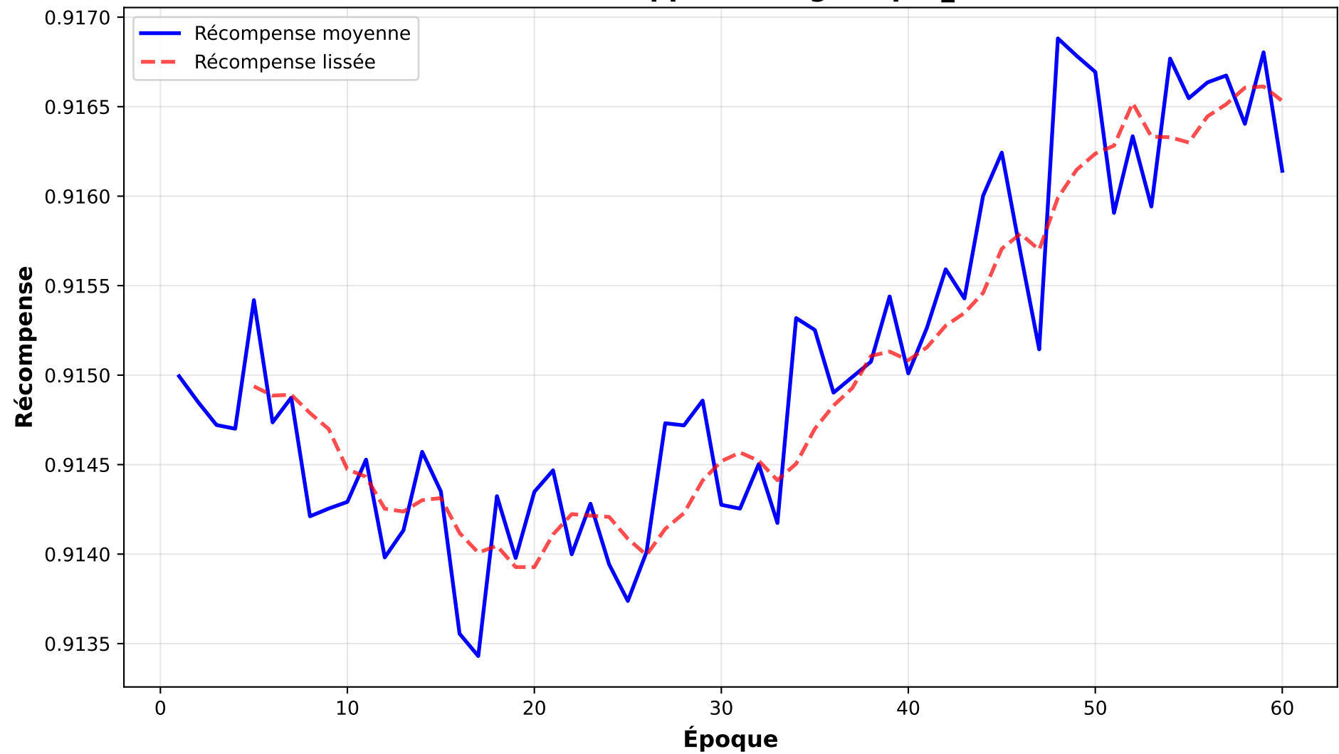
Courbe d'apprentissage - split_3
