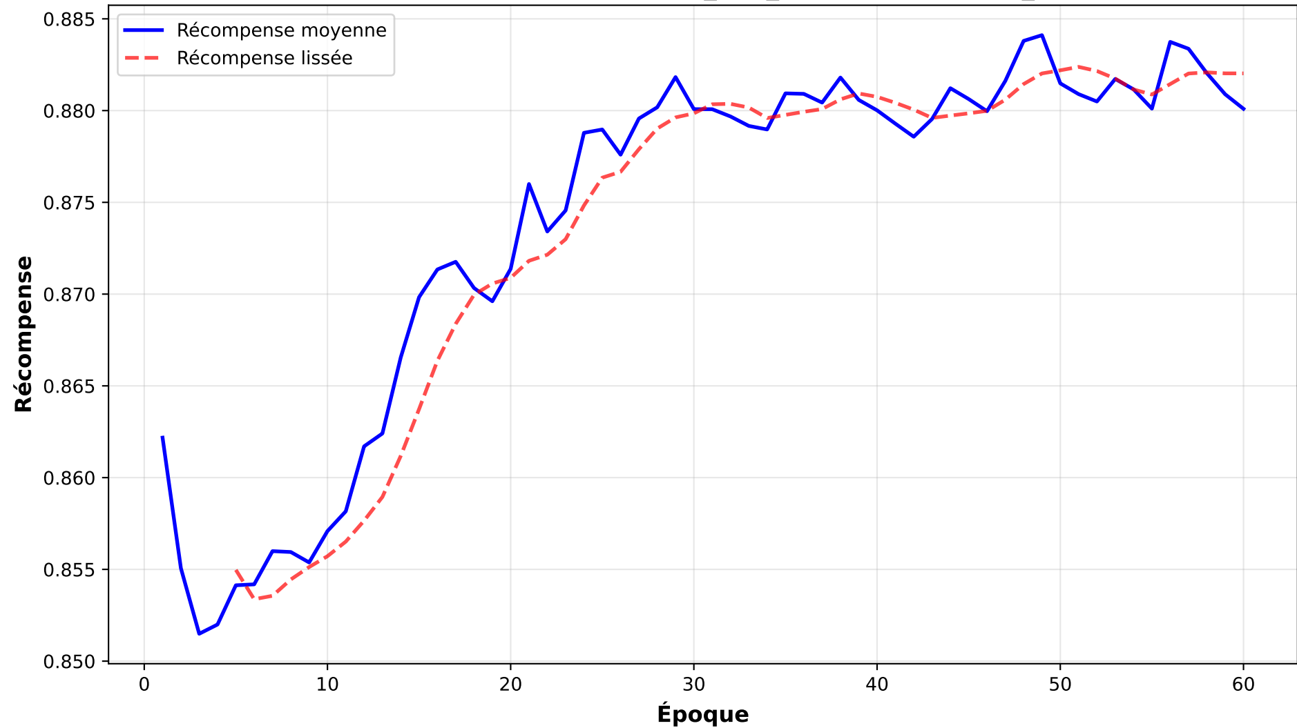
Courbe d'apprentissage - alt_run_dhash-optimized_split2
