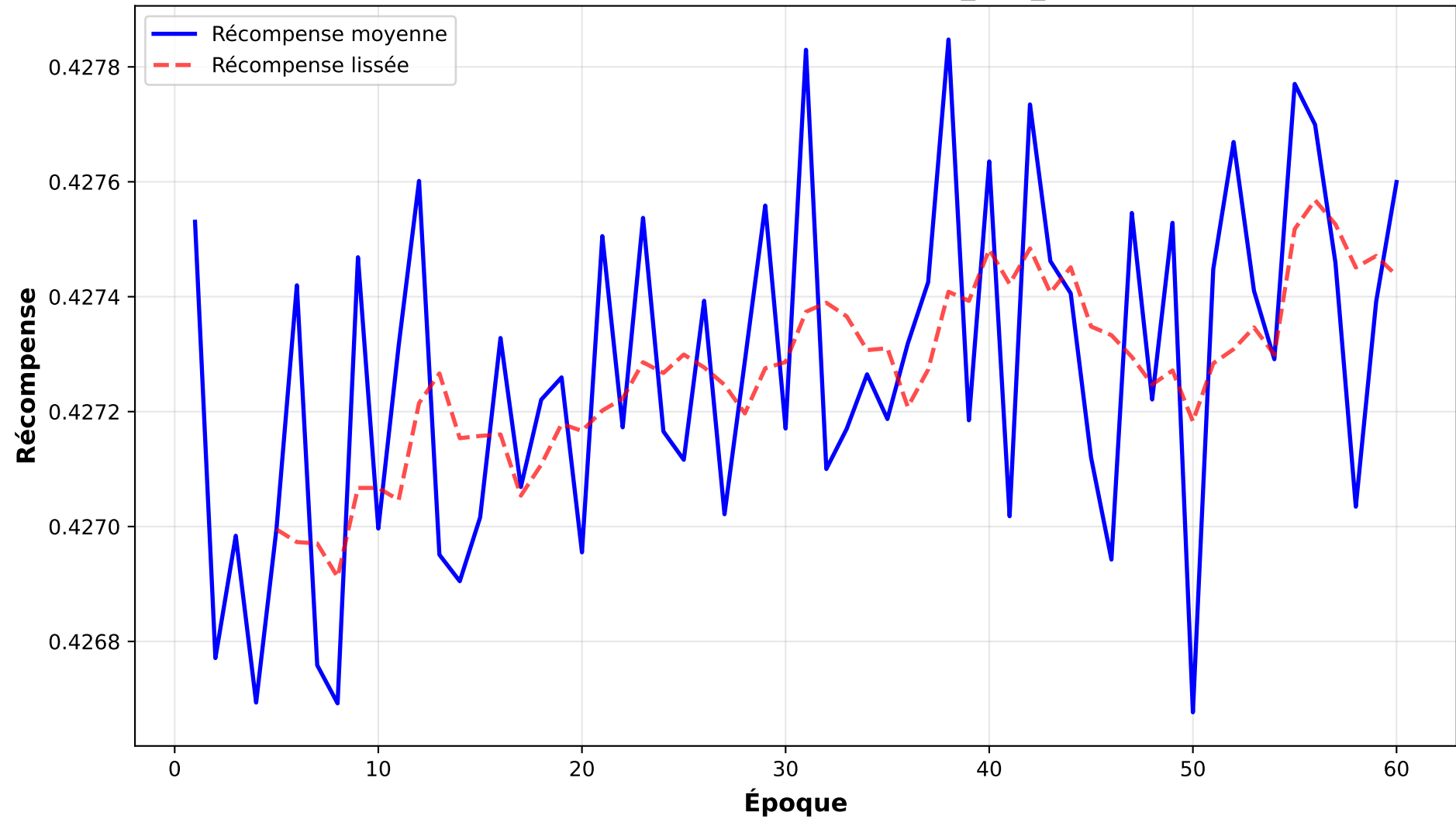
Courbe d'apprentissage - alt_run_kts
