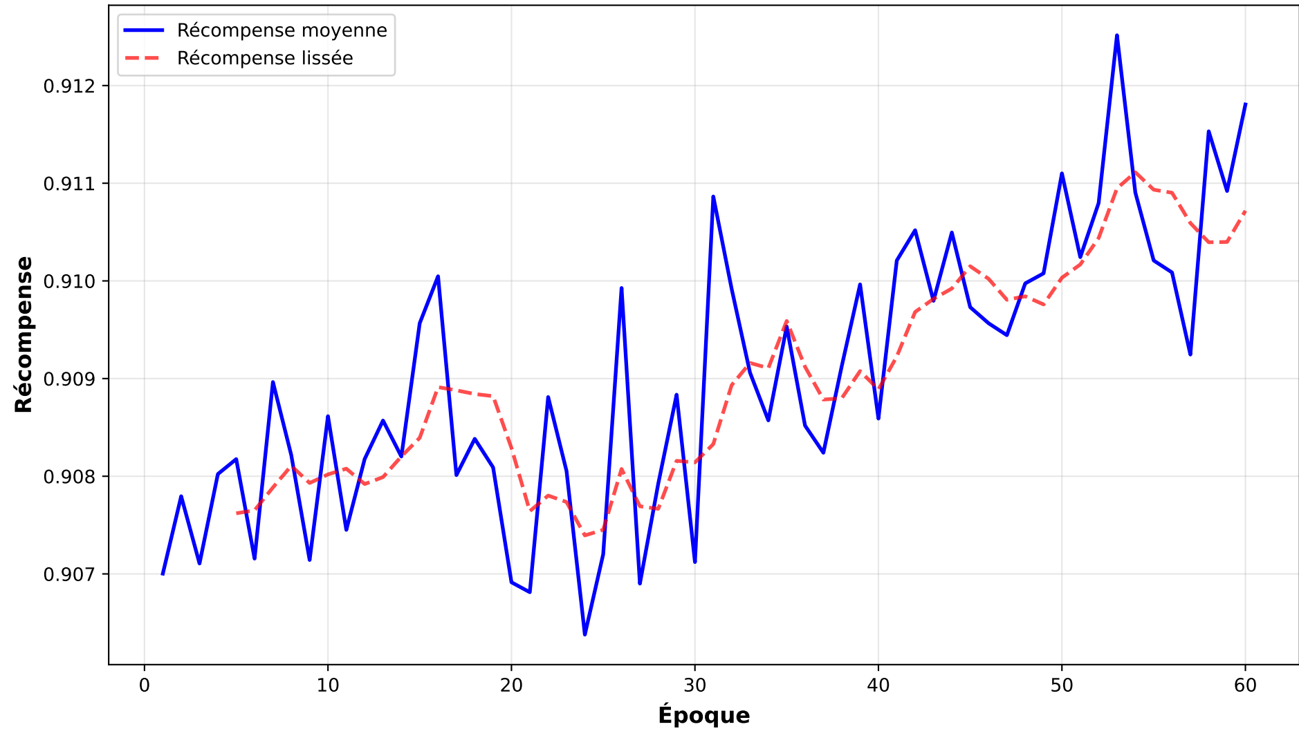
Courbe d'apprentissage - R-DSN-summe-split3
