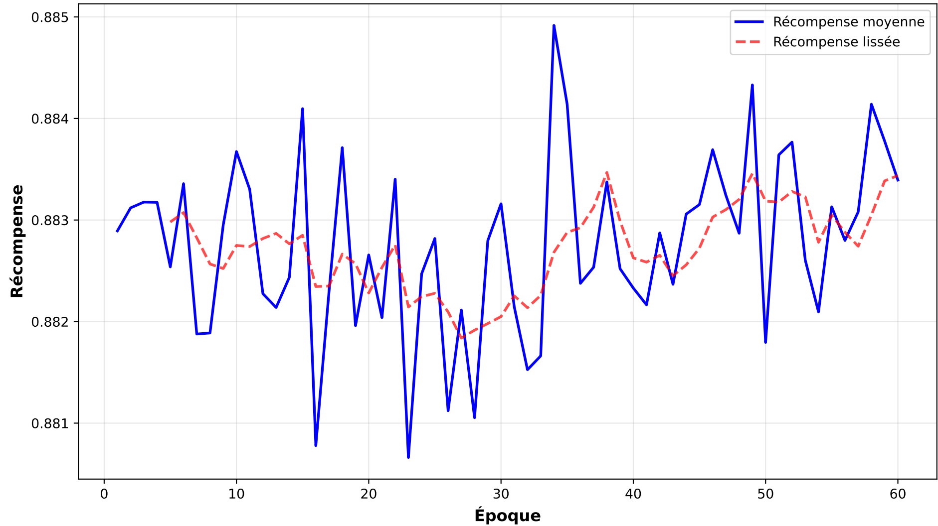
Courbe d'apprentissage - DR-DSN-summe-split1
