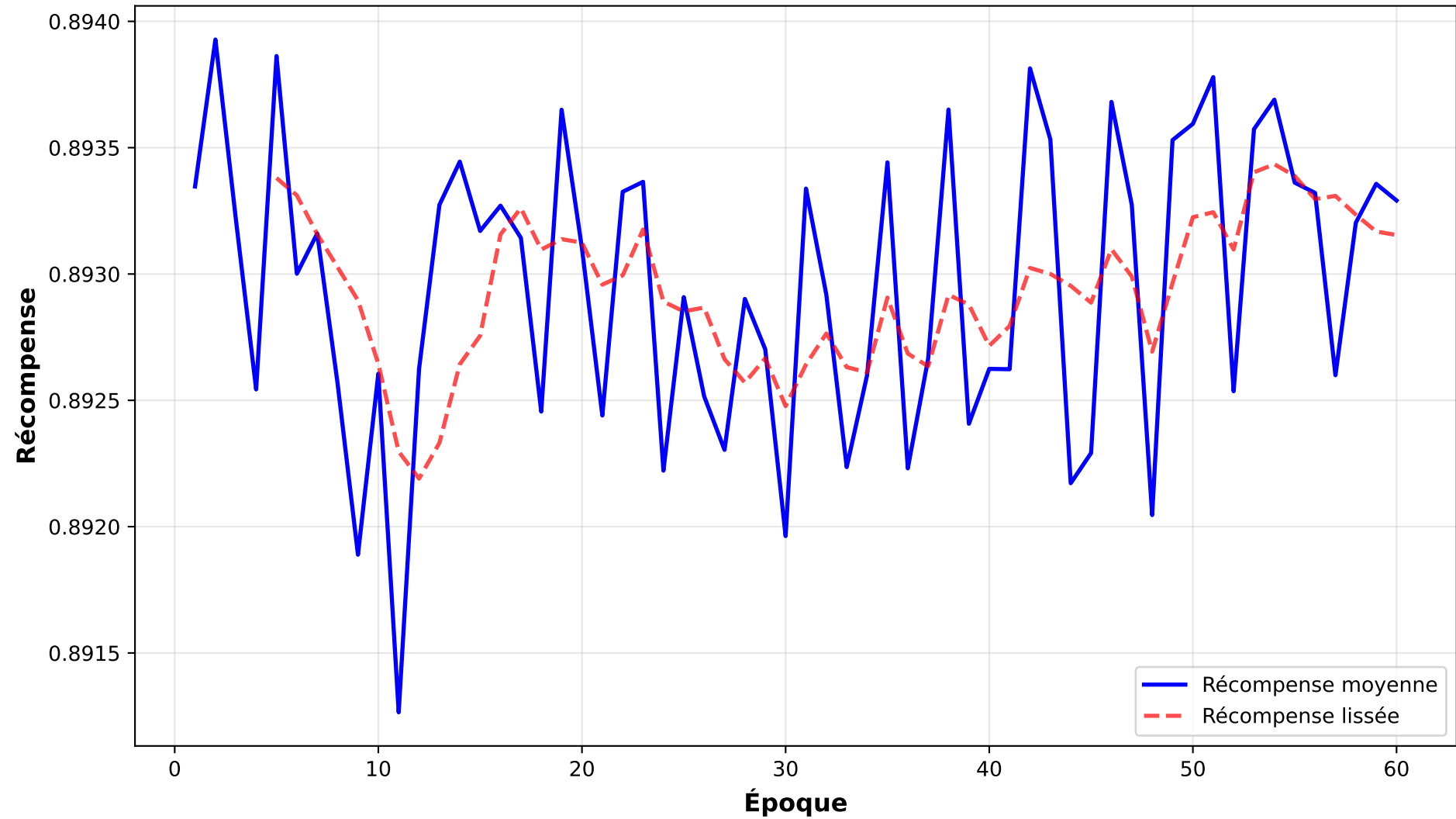
Courbe d'apprentissage - DR-DSN-summe-split3
