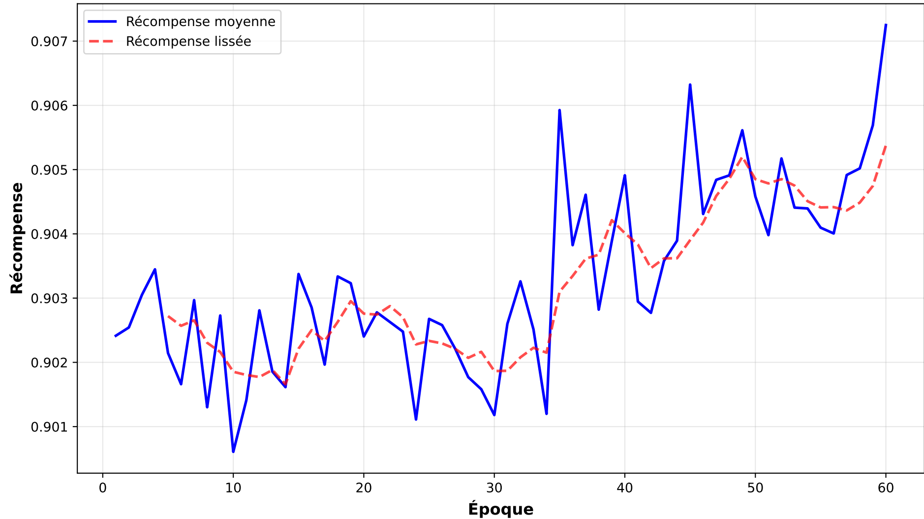
Courbe d'apprentissage - R-DSN-summe-split4
