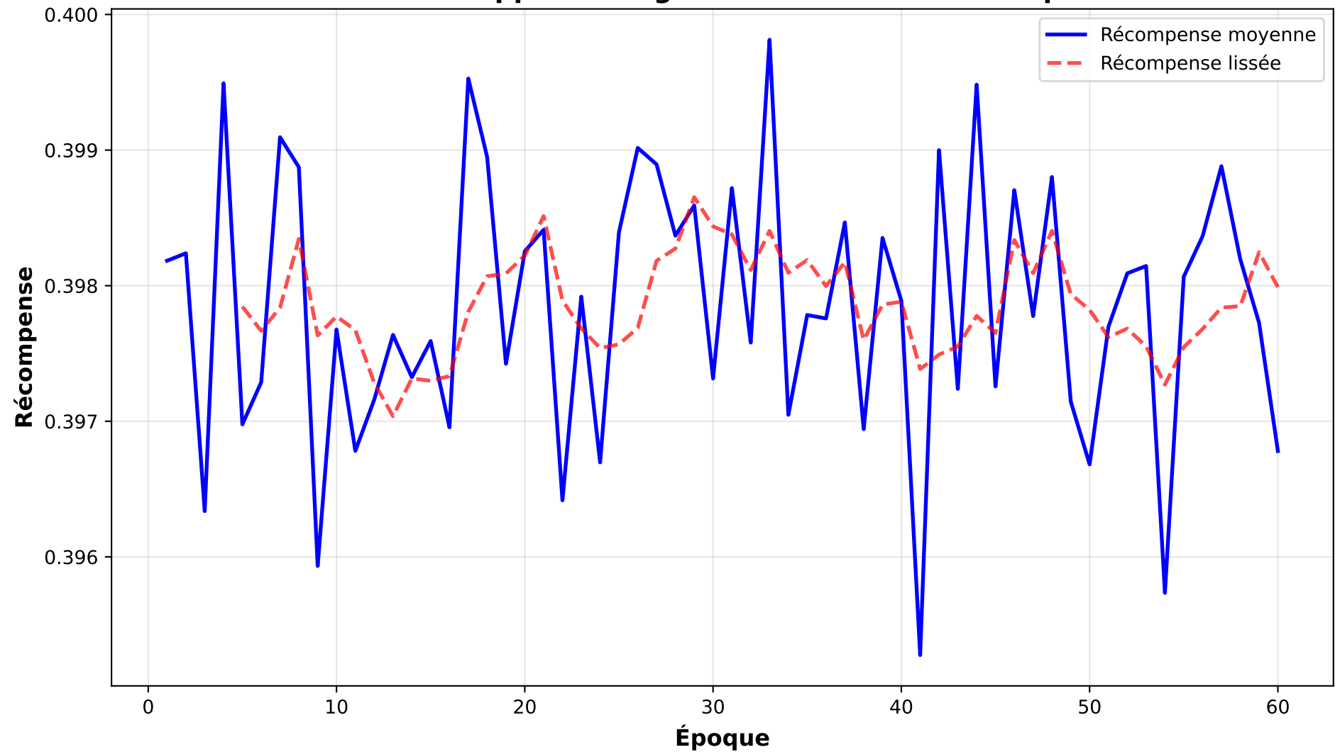
Courbe d'apprentissage - d-nolambda-summe-split3
