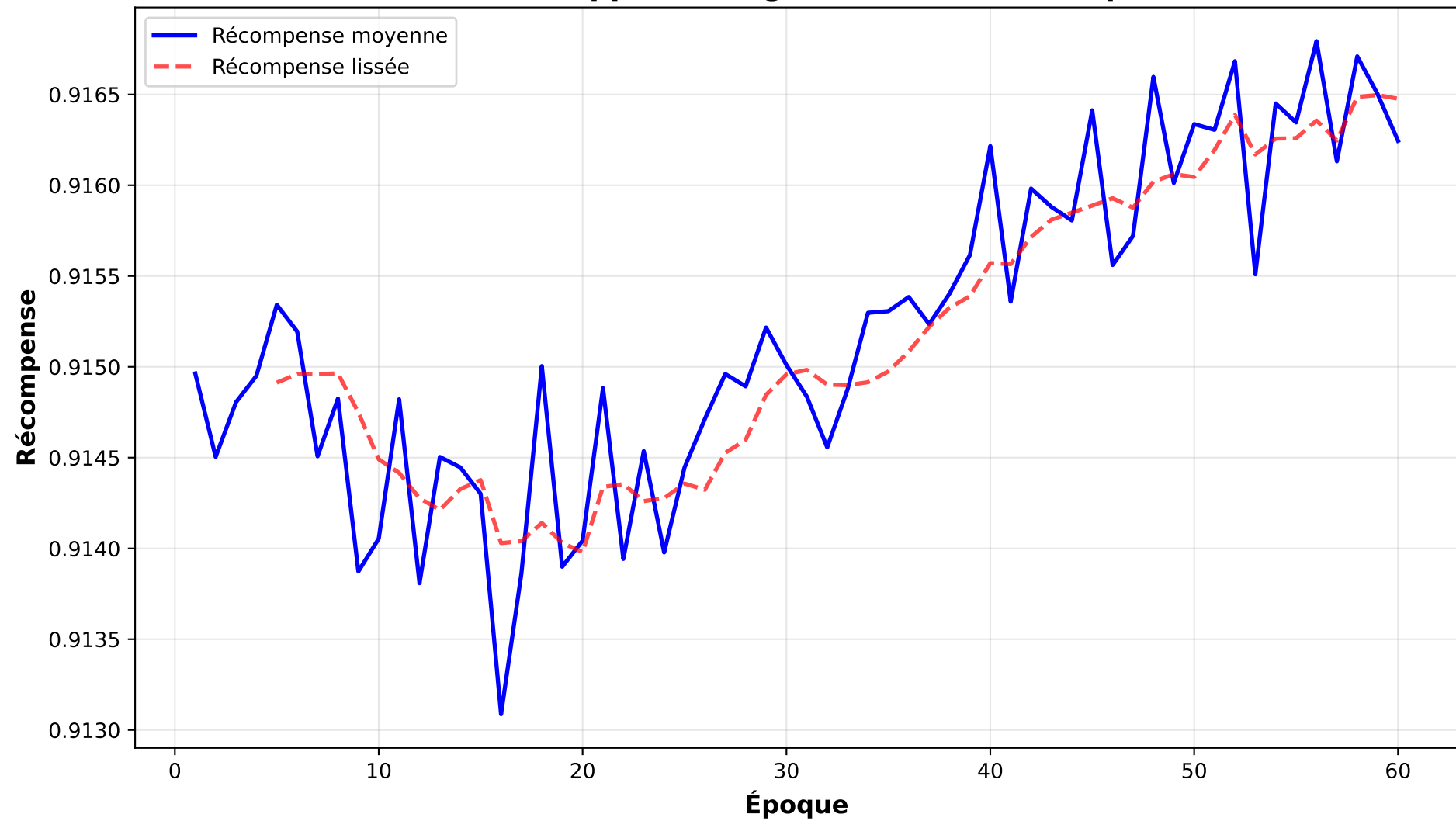
Courbe d'apprentissage - DR-DSN-tvsum-split3
