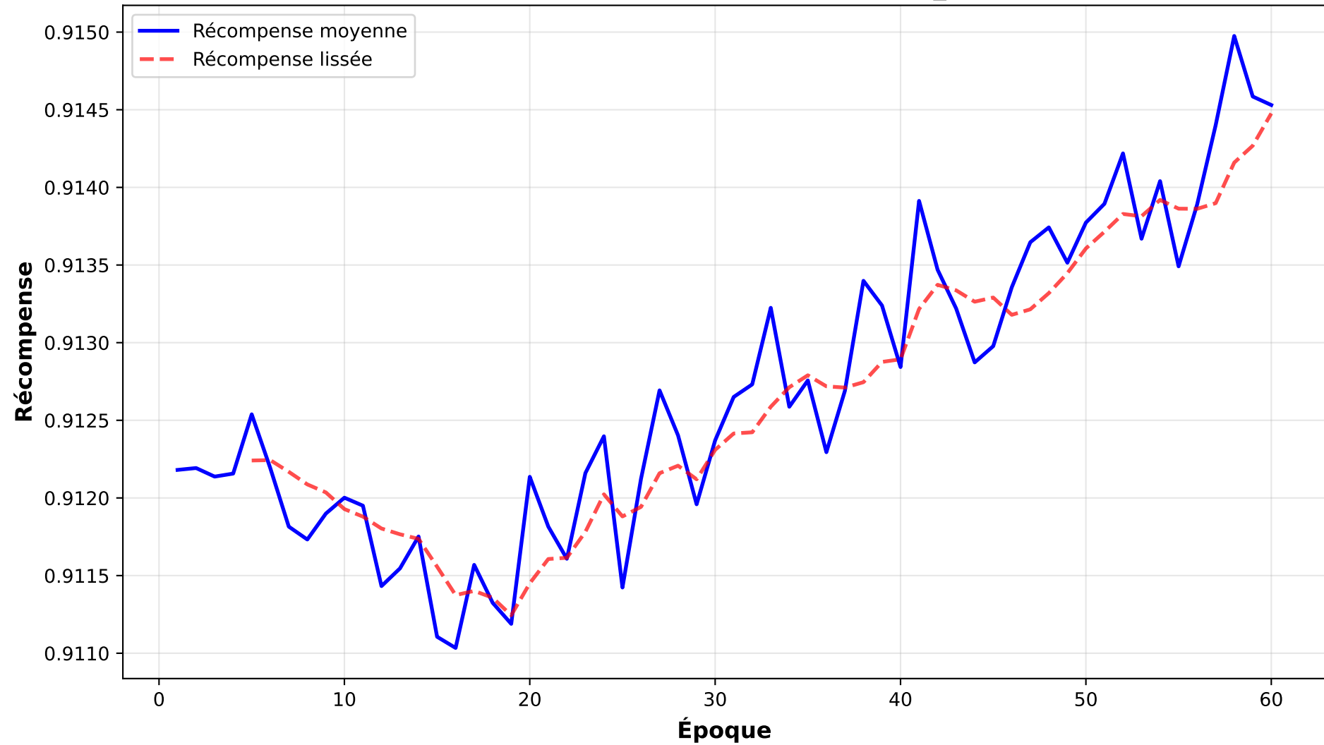
Courbe d'apprentissage - split_2
