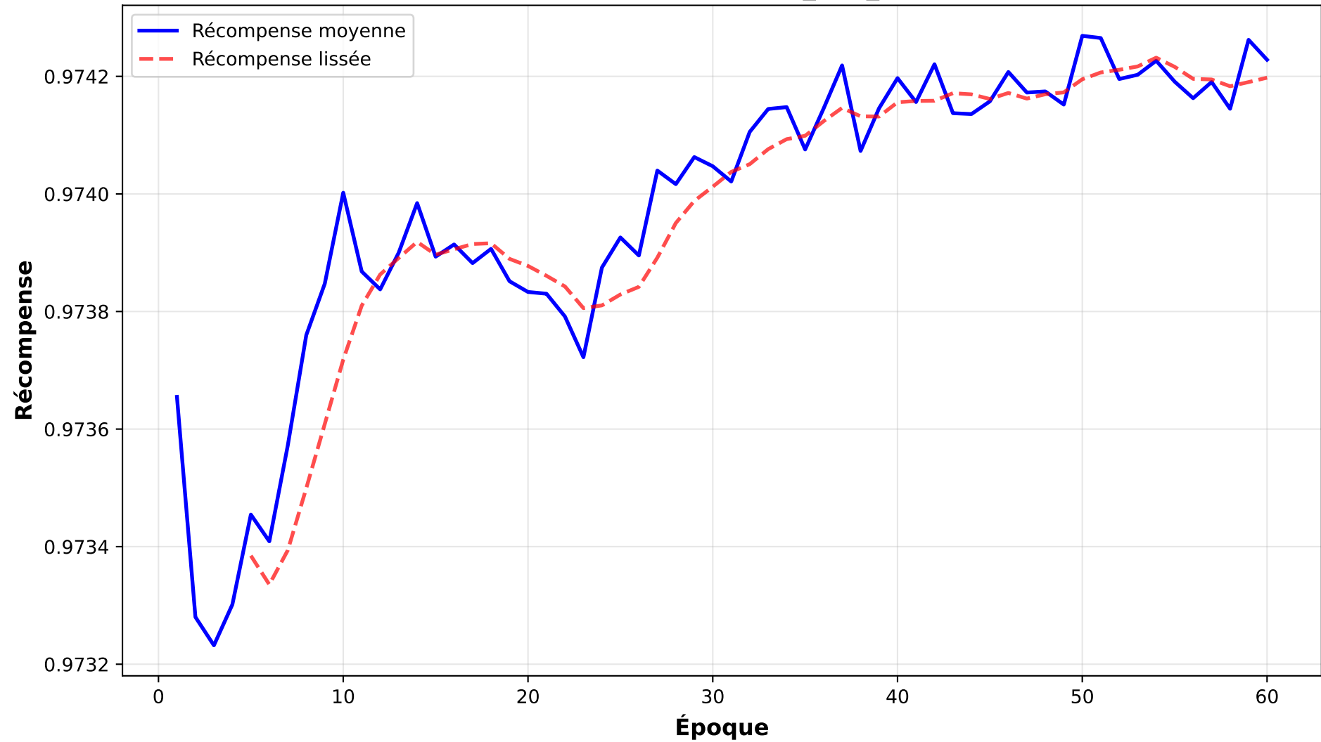
Courbe d'apprentissage - alt_run_dhash-split0
