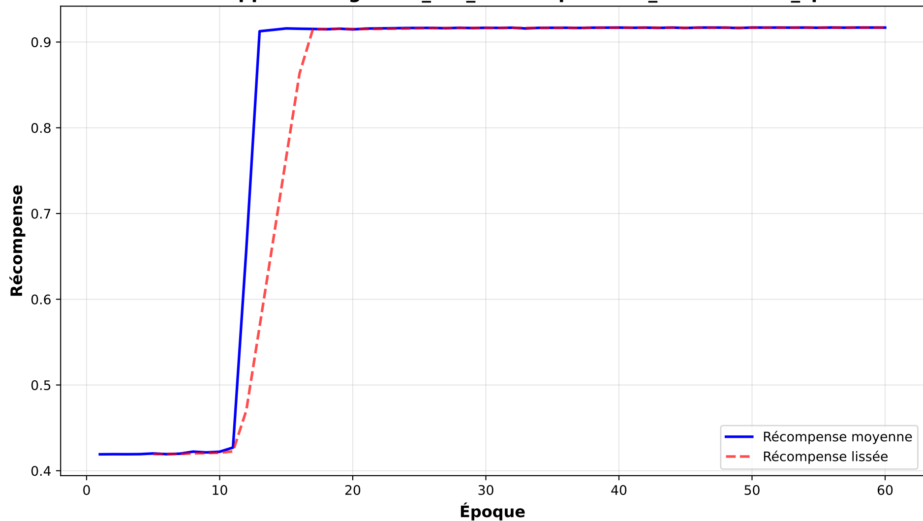
Courbe d'apprentissage - alt_run_dhash-optimized_newFeatures_split0
