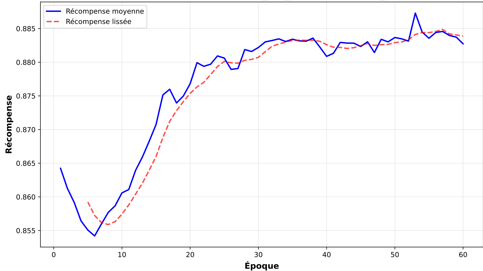
Courbe d'apprentissage - alt_run_dhash-optimized_split3
