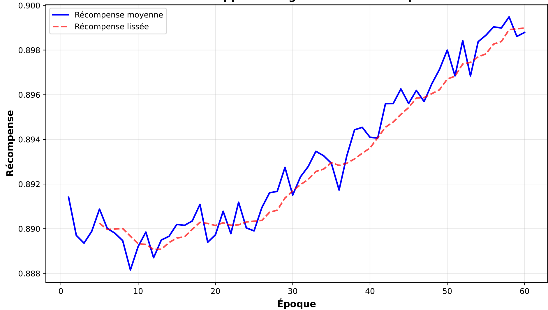
Courbe d'apprentissage - R-DSN-tvsum-split3
