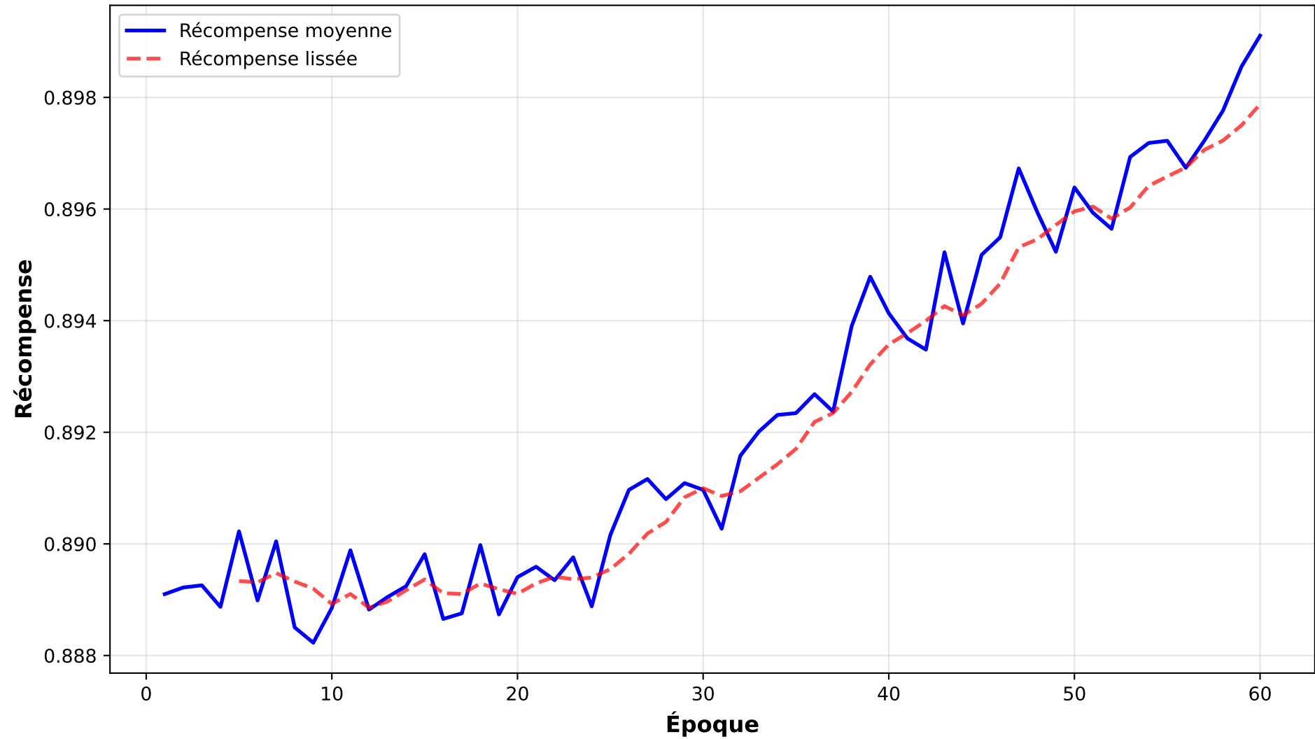
Courbe d'apprentissage - R-DSN-tvsum-split4
