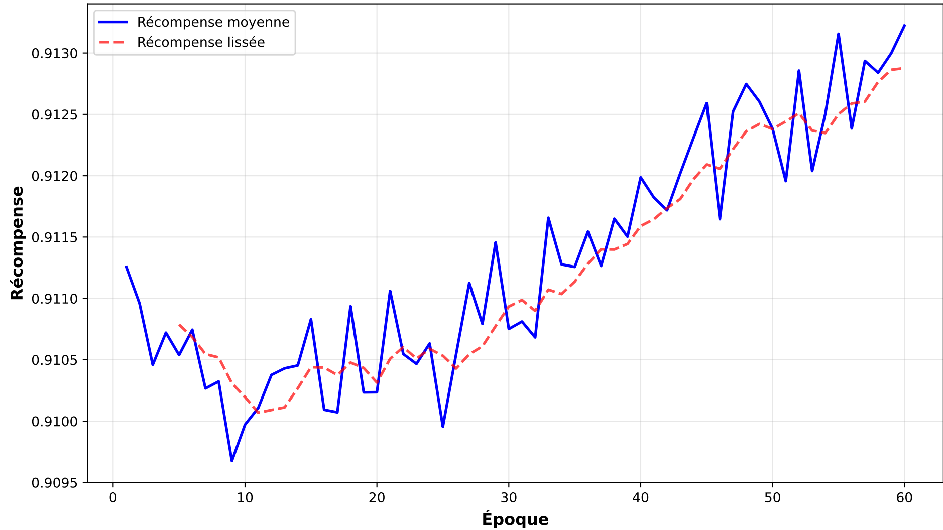
Courbe d'apprentissage - DR-DSN-tvsum-split0
