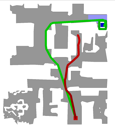
IEVE
