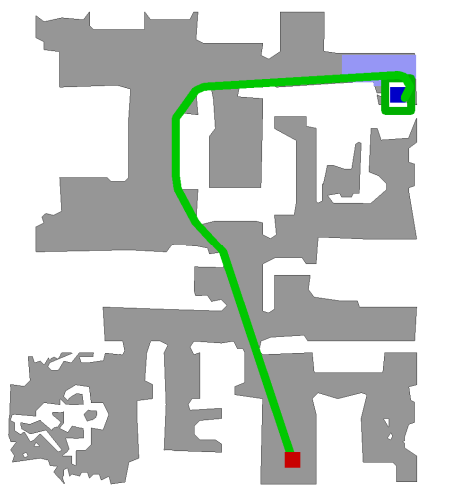
GaussNav
